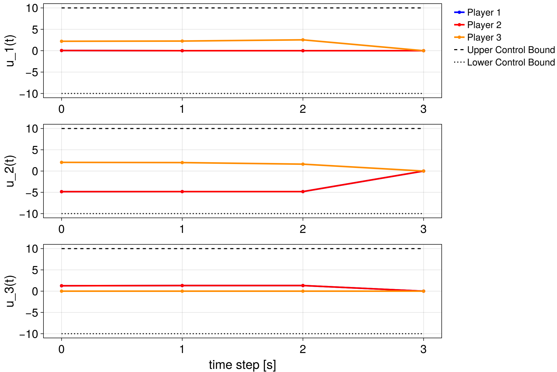
MPC step 2/3
