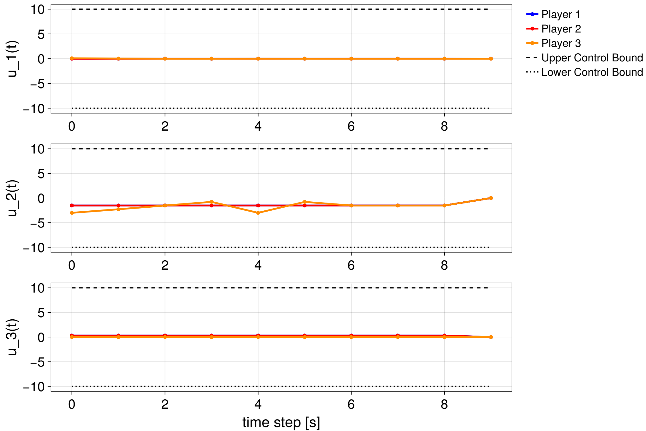
MPC step 24/30
