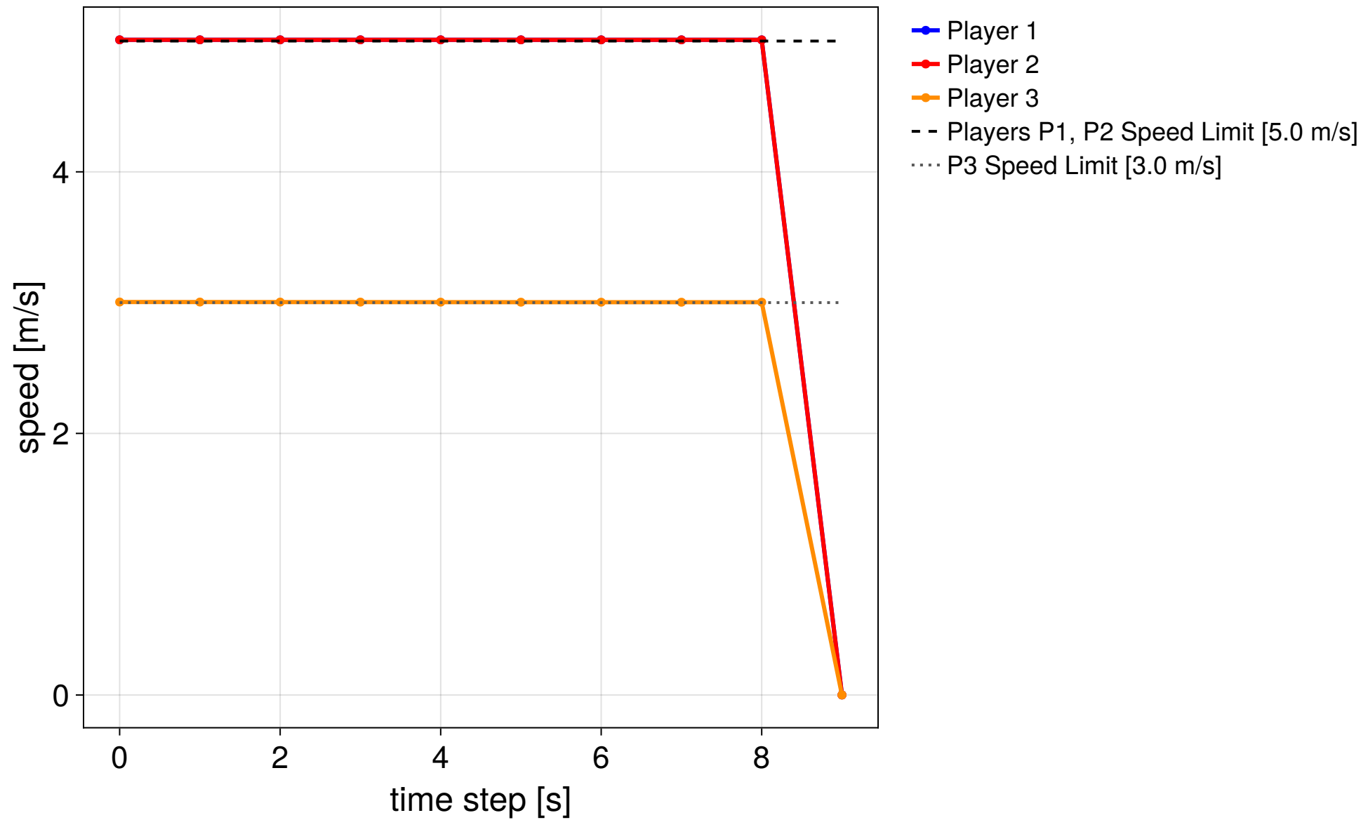
MPC step 7/30
