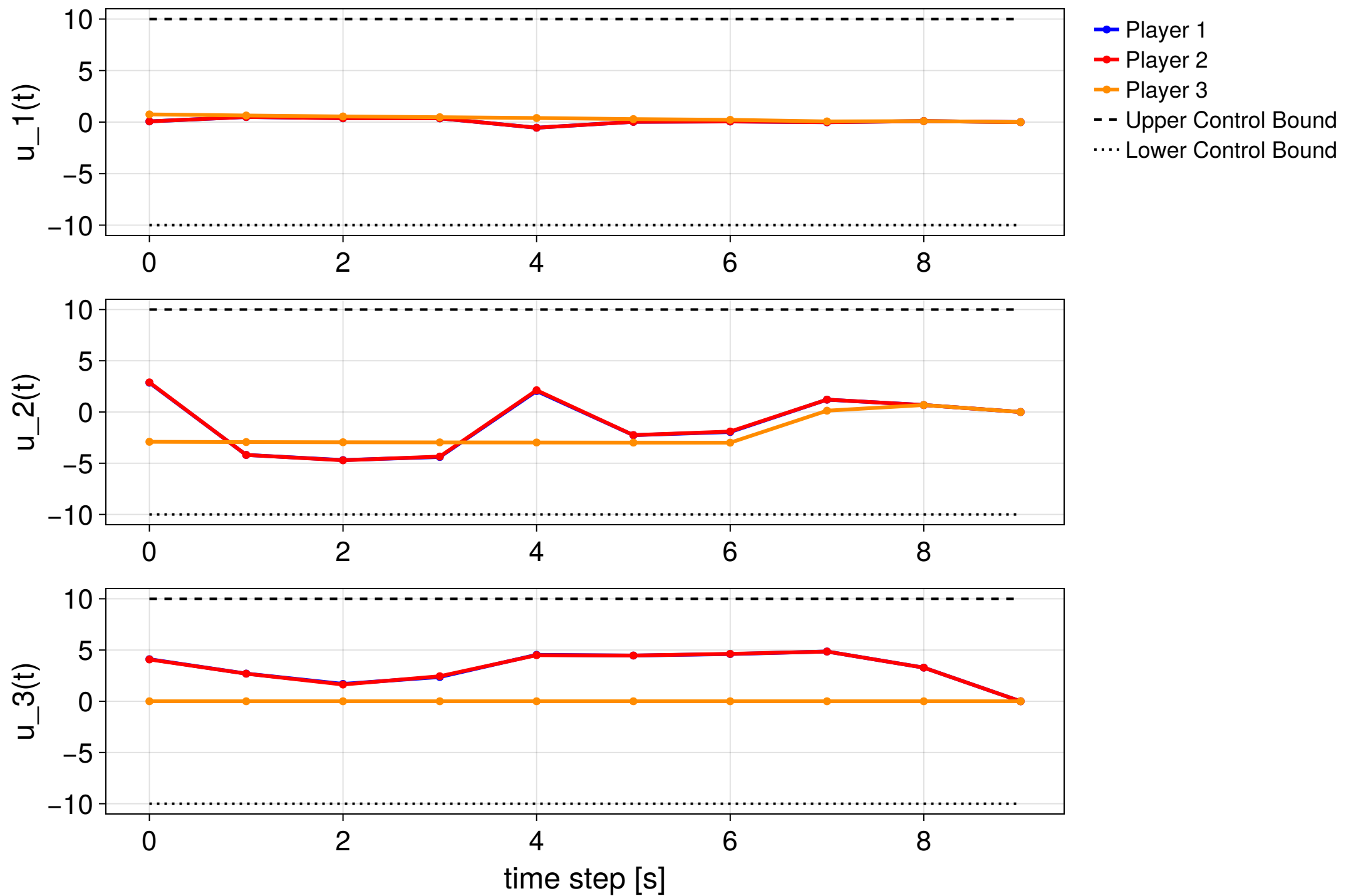
MPC step 23/30
