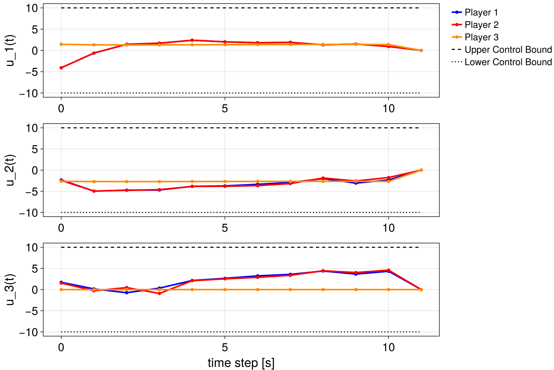
MPC step 15/25 — NOT CONVERGED (KKT error 0.154)
