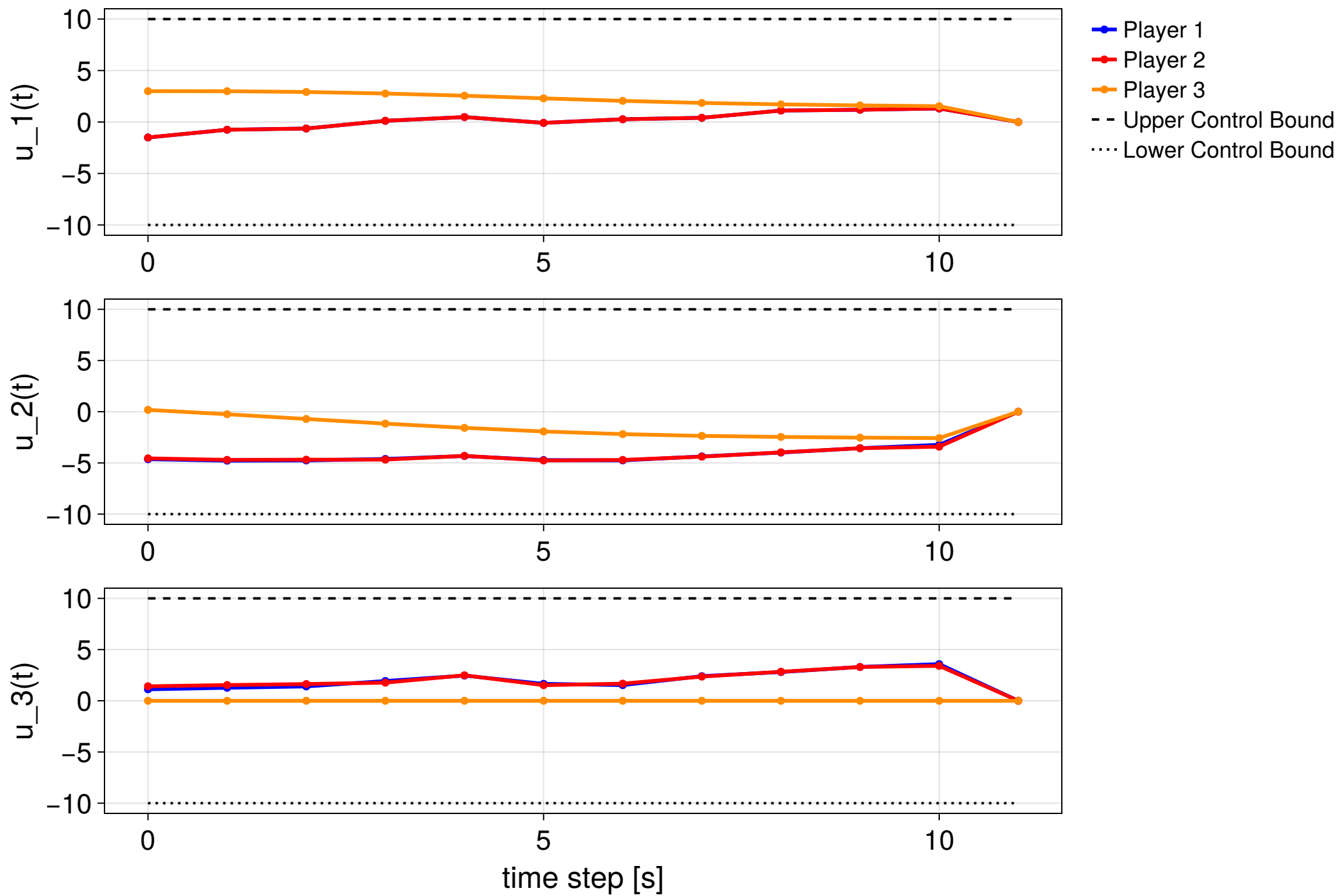
MPC step 9/25
