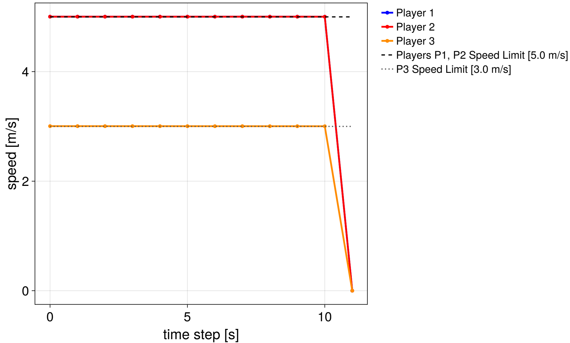
MPC step 2/25
