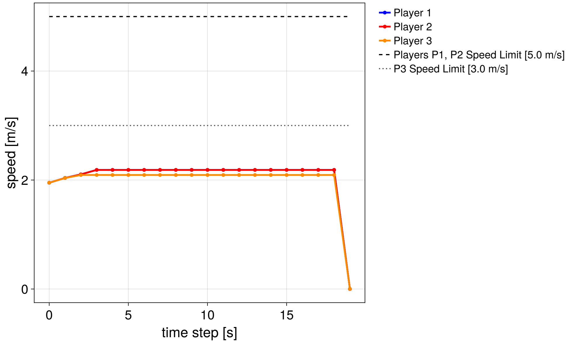
MPC step 22/30
