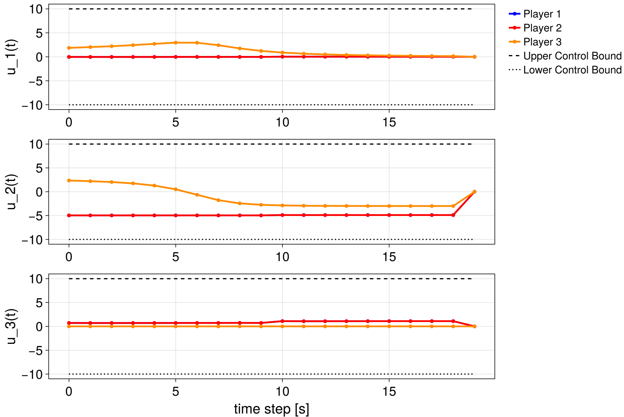
MPC step 3/30
