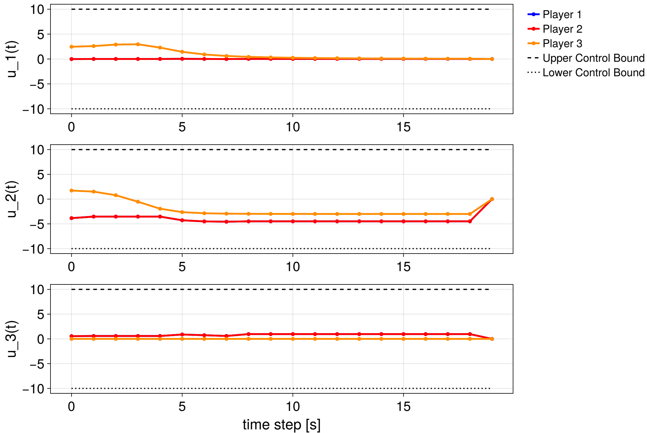
MPC step 7/30
