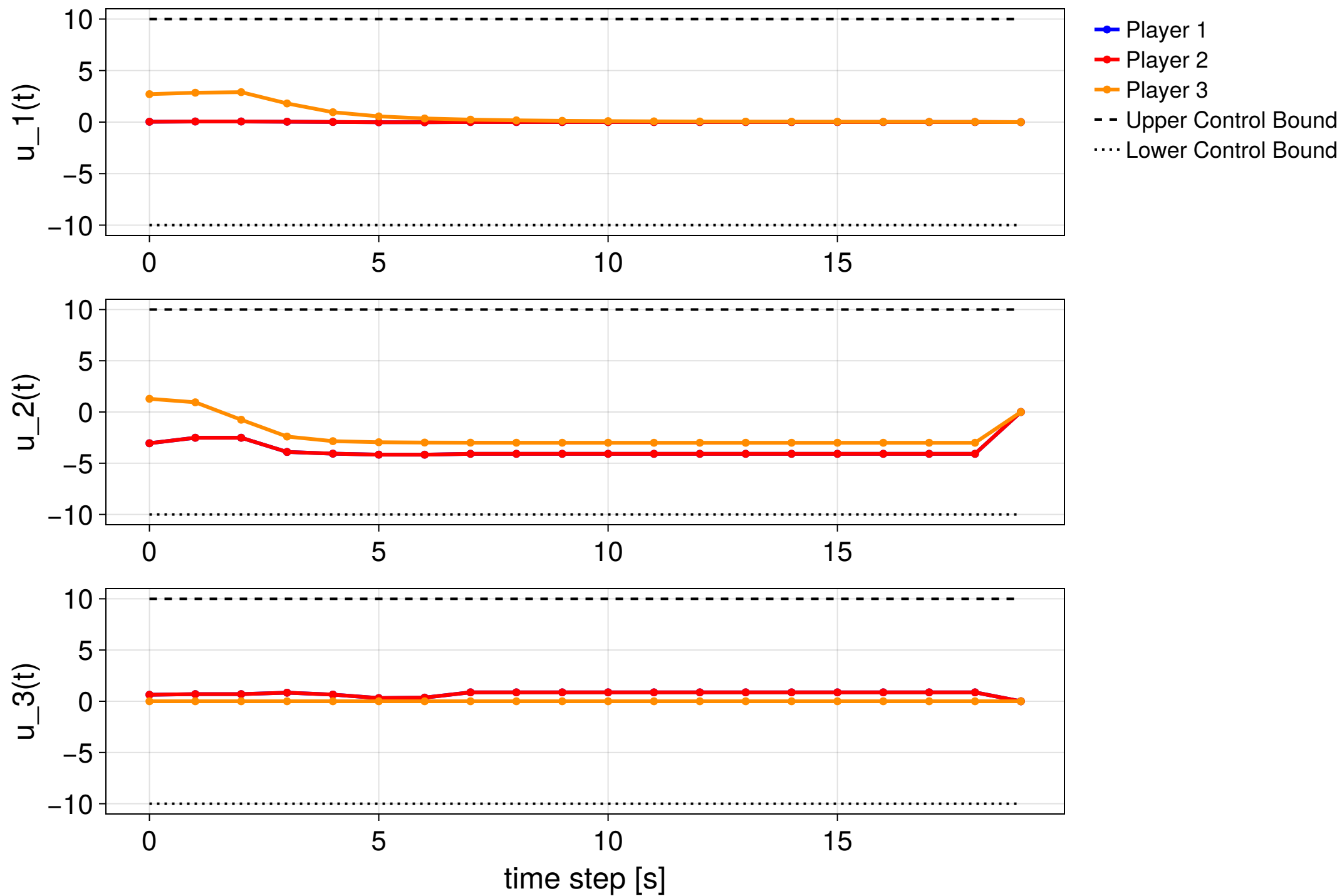
MPC step 9/30
