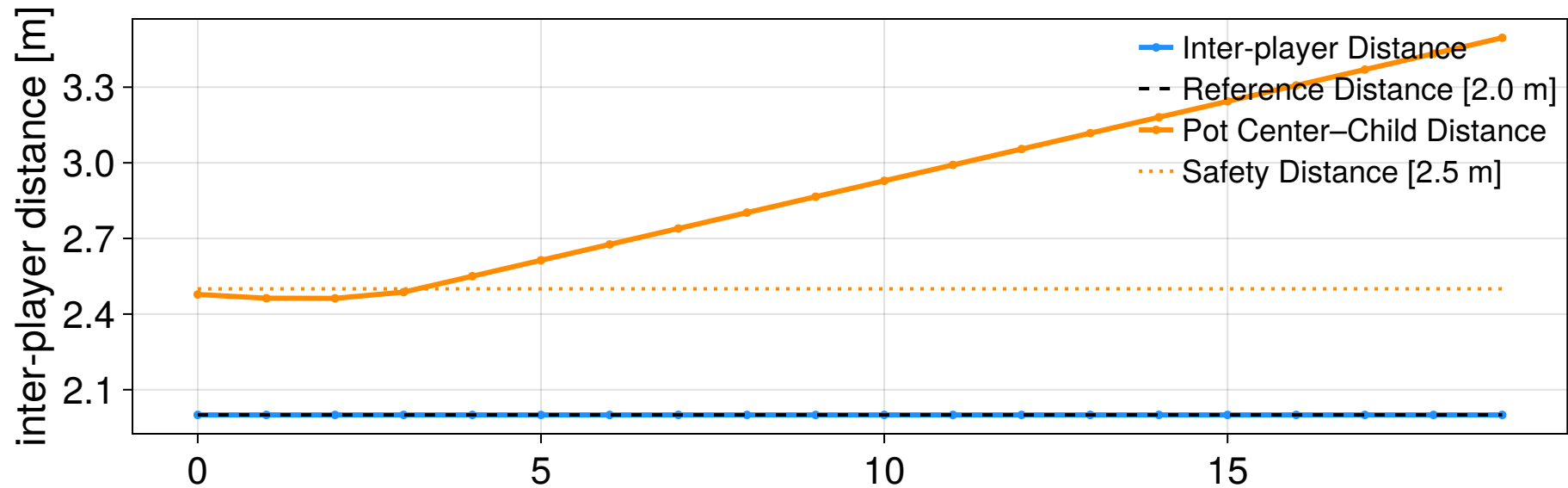
MPC step 24/30
