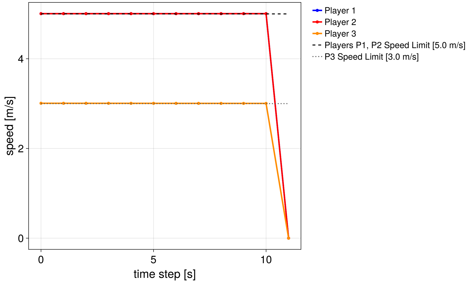
MPC step 2/20
