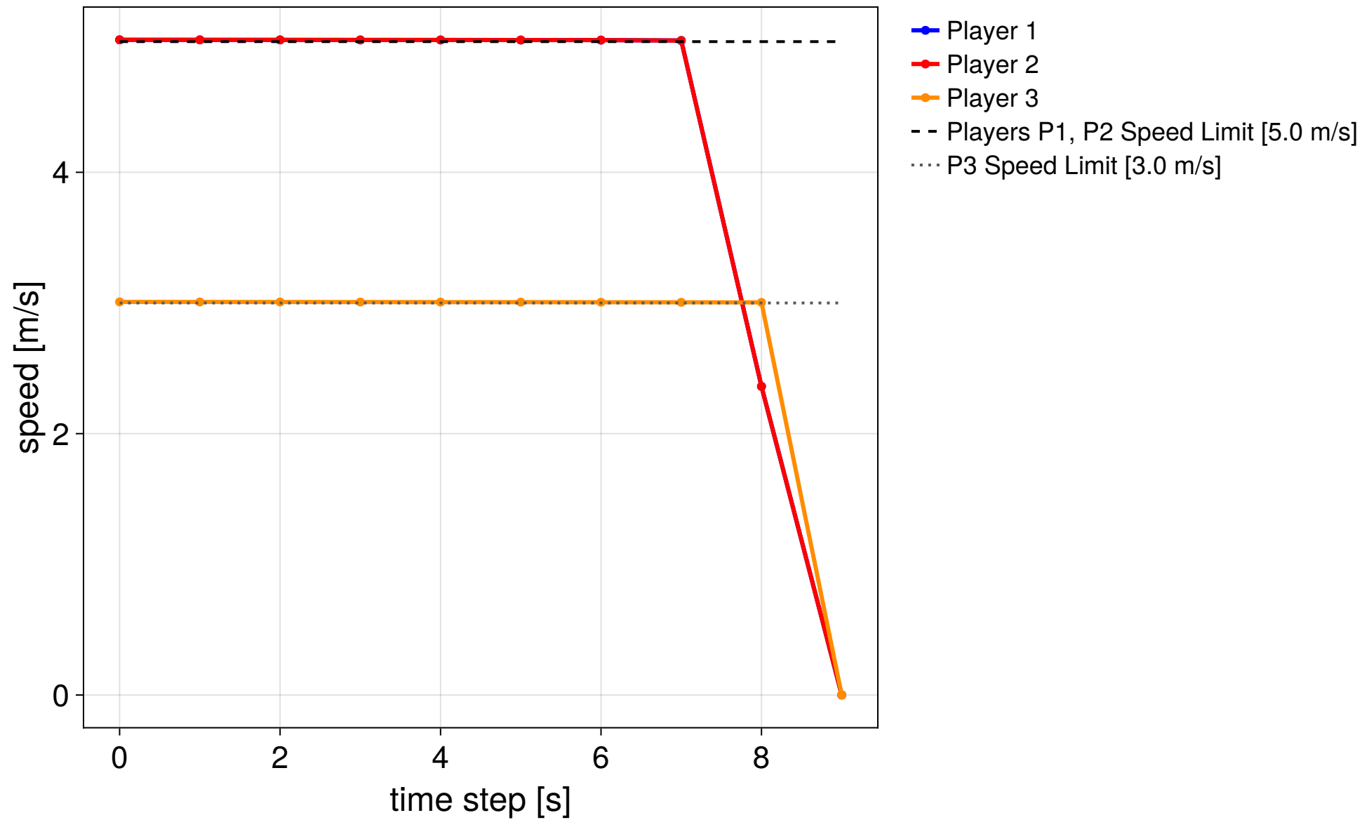
MPC step 1/2
