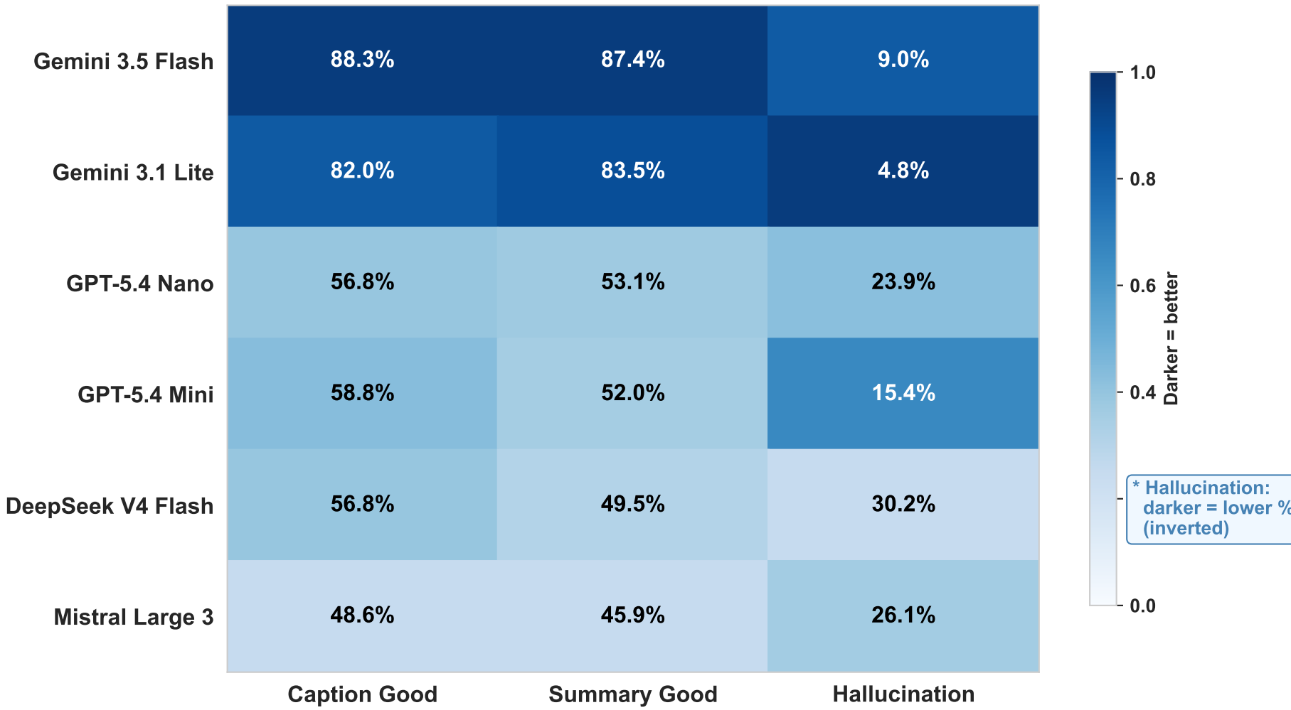
(d) Overall Heatmap
