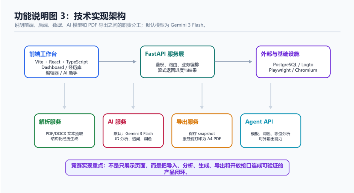
图 3 技术实现架构：展示前端、FastAPI 后端、数据层、默认 AI 模型 Gemini 3 Flash 与导出服务的职责分工。
