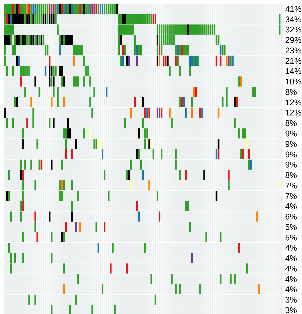
LUAD-ROY (N = 137)
