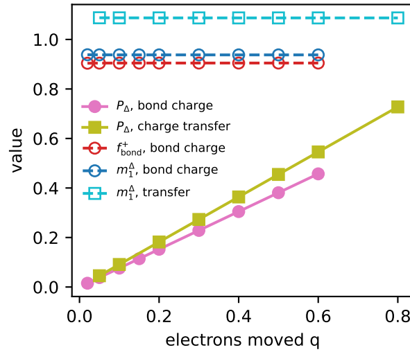
(d) only the polarity scales with q
