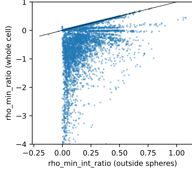
(d) whole cell vs interstitial (Spearman 0.36)
