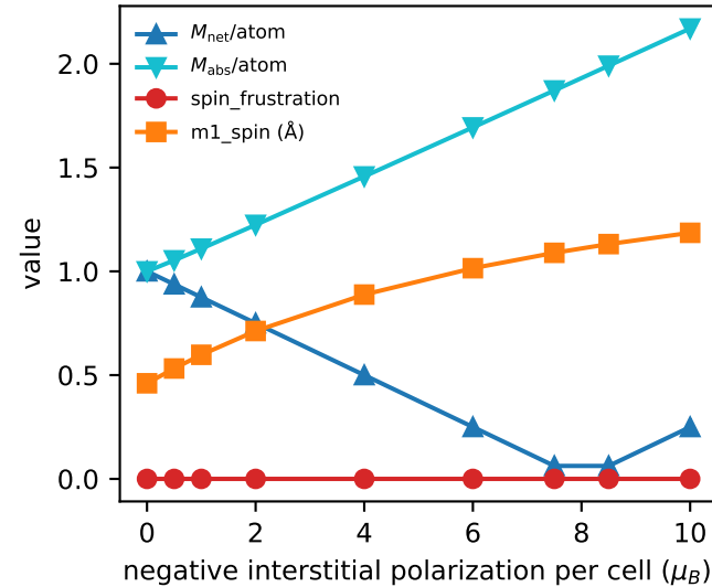
(d) FM + antiparallel interstitial spin
