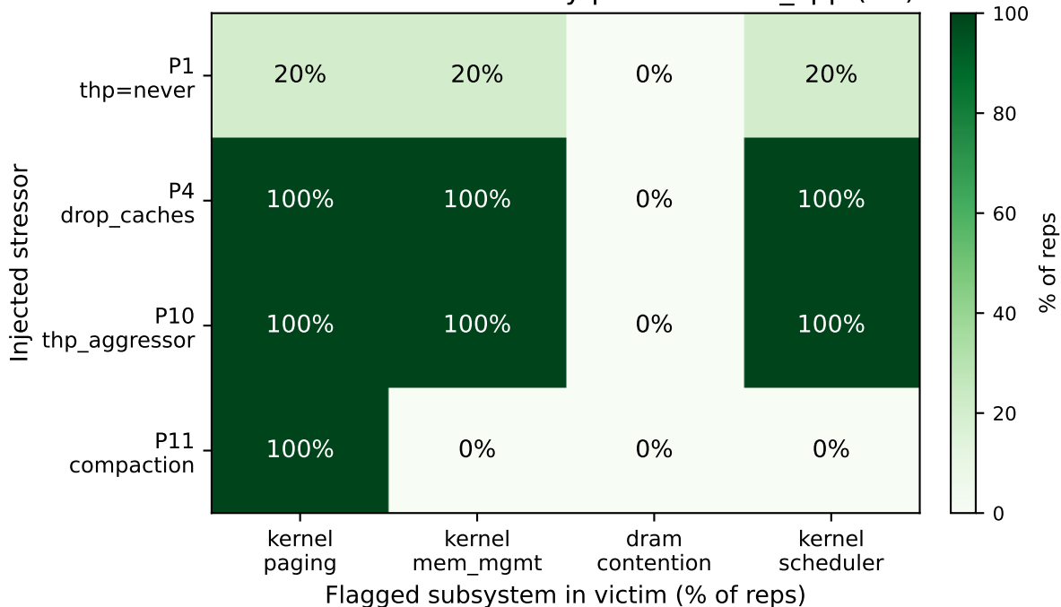
Victim-Mode vulnerability profile: llama_cpp (B0)
