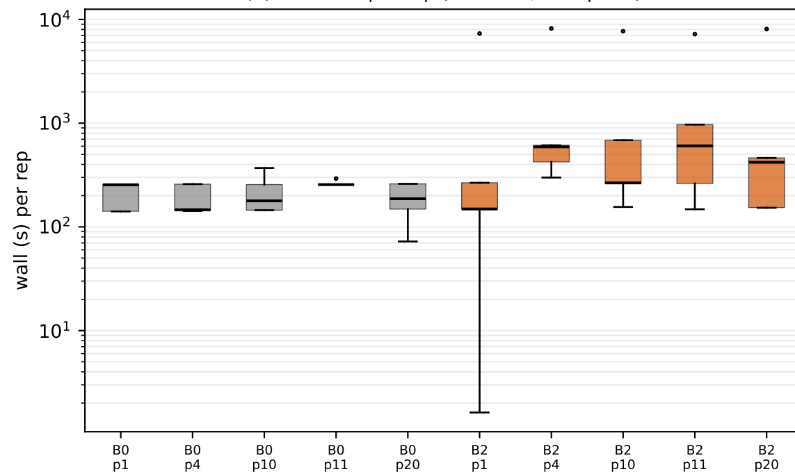
(d) wall time per rep (B0 vs B2, all 5 perts)
