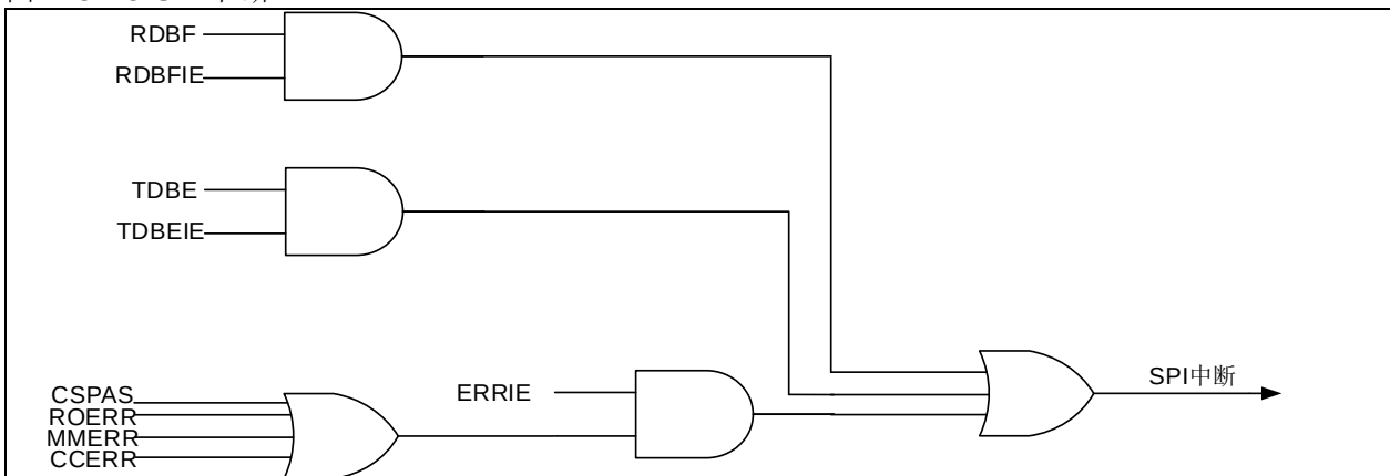
图 13-18 SPI中断
