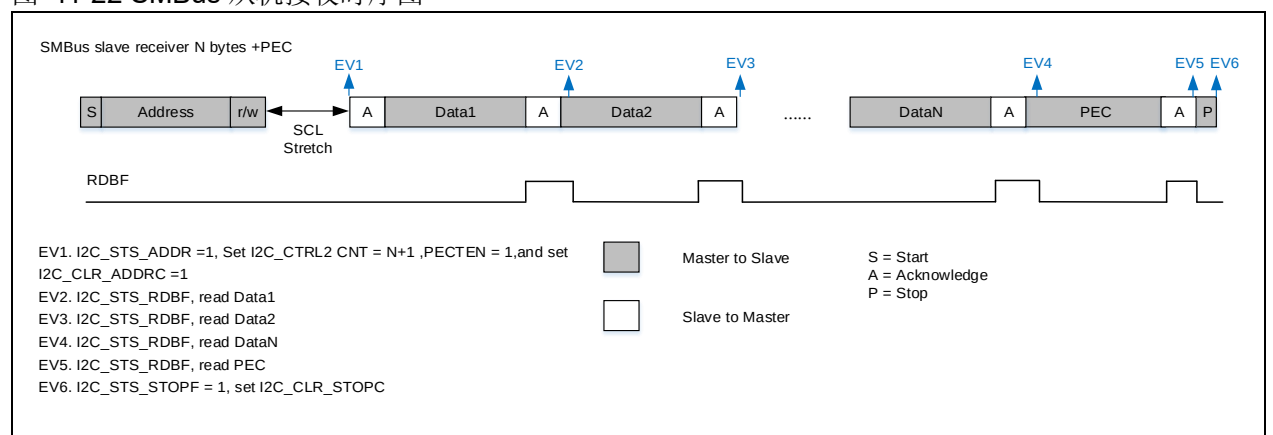
图 11-22 SMBus 从机接收时序图
