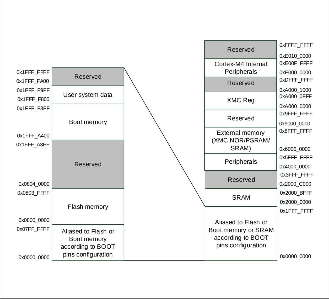
图 2-1 AT32F423地址配置
