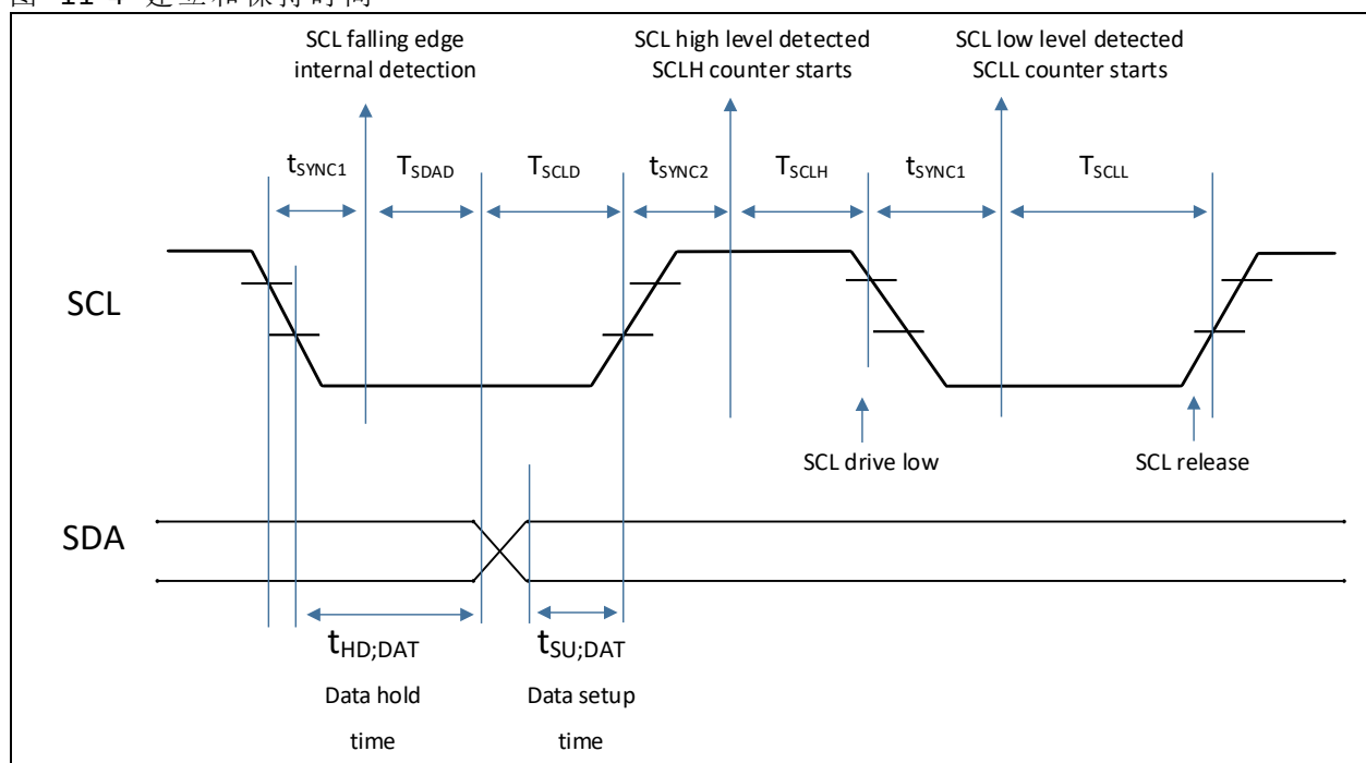
图 11-4 建立和保持时间
