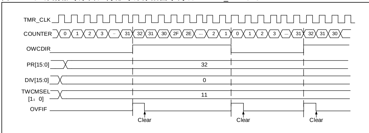
图 14-48 计数器时序图，内部时钟分频因子为0，TMRx_PR=0x32
