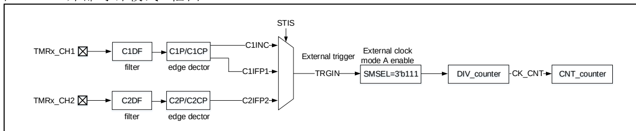
图 14-41 外部时钟模式 A 框图
