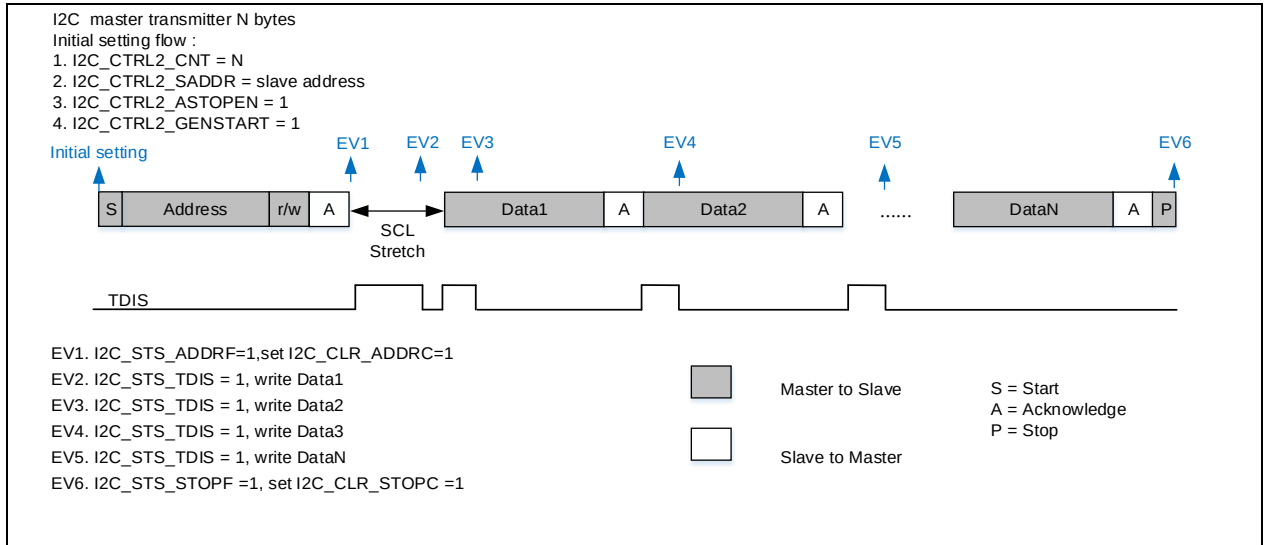
图 11-6 I 2 C主机发送时序图
