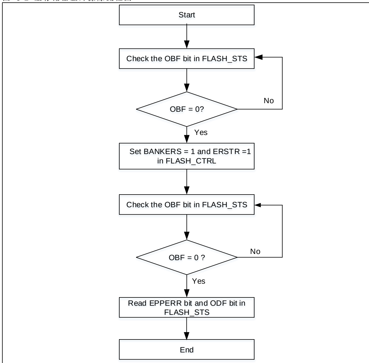
图 5-2 主存储器整片擦除流程图
