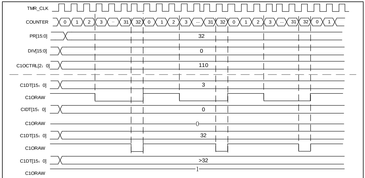
图 14-27 向上计数下 PWM 模式 A
