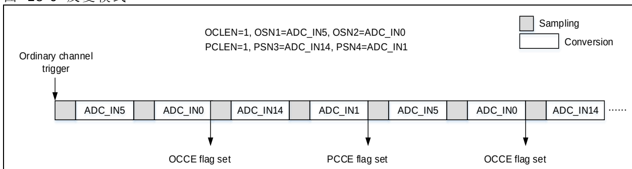
图 18-6 反复模式
