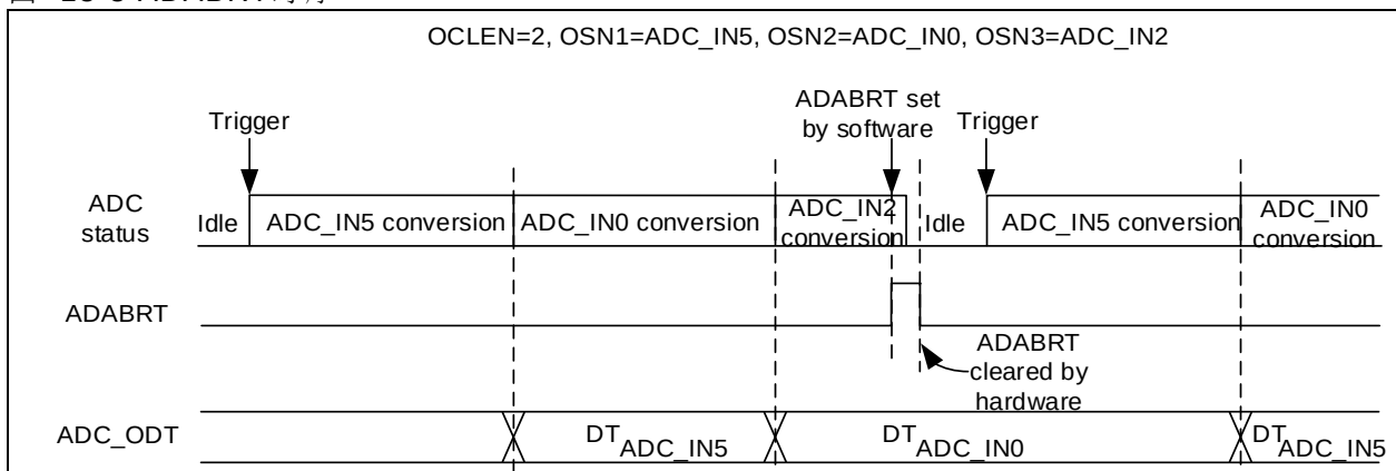
图 18-8 ADABRT 时序
