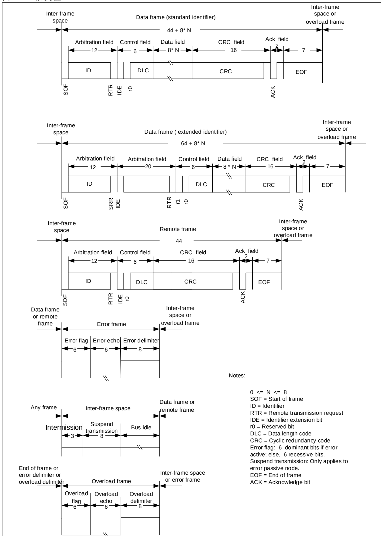
图 20-2帧类型
