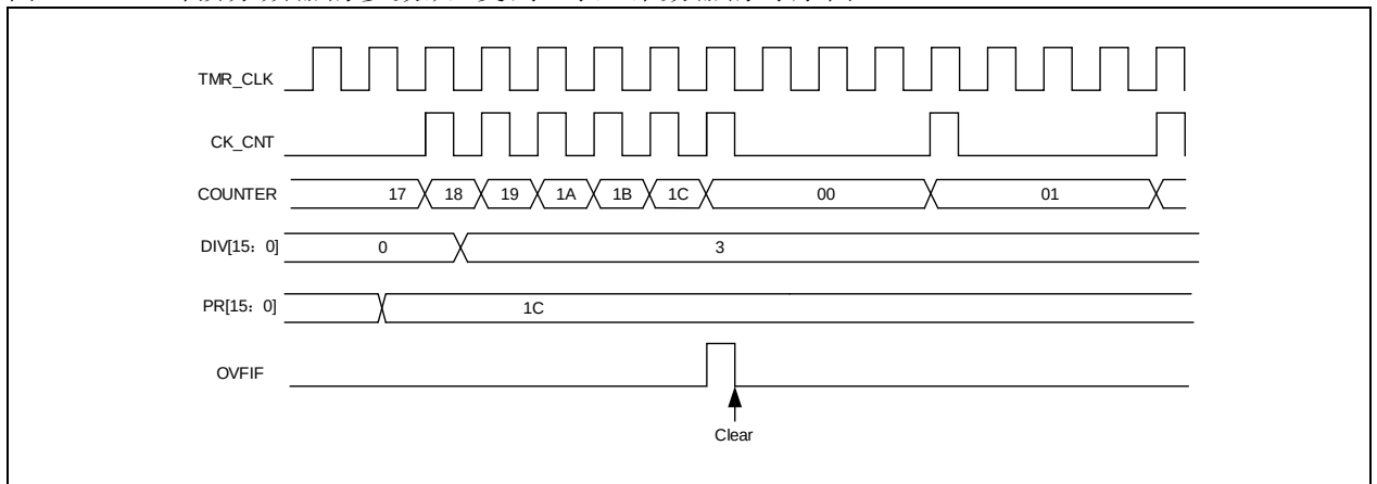
图 14-90 当预分频器的参数从0变到3时，计数器的时序图
