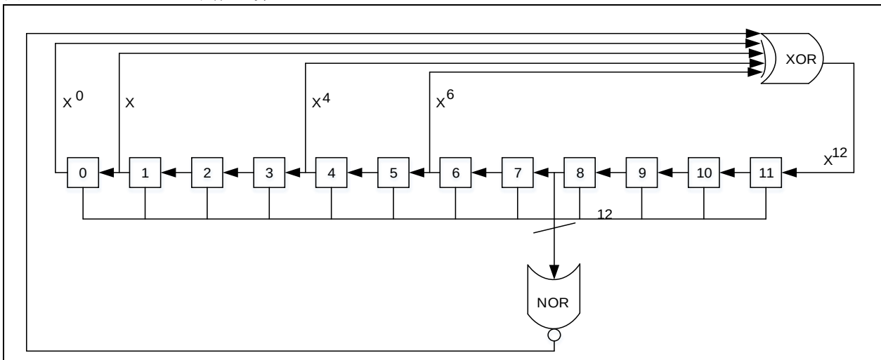
图 19-2 DAC LFSR寄存器算法
