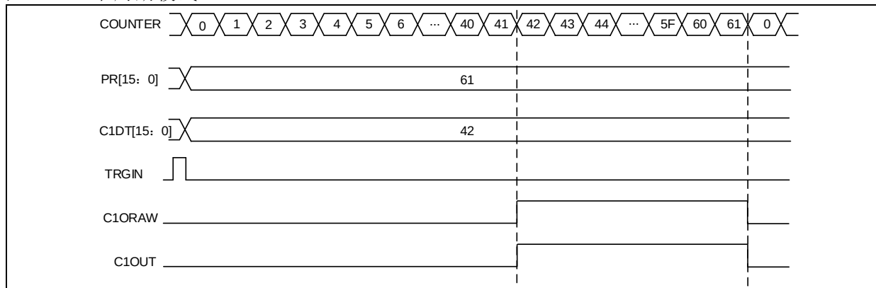
图 14-58 单周期模式
