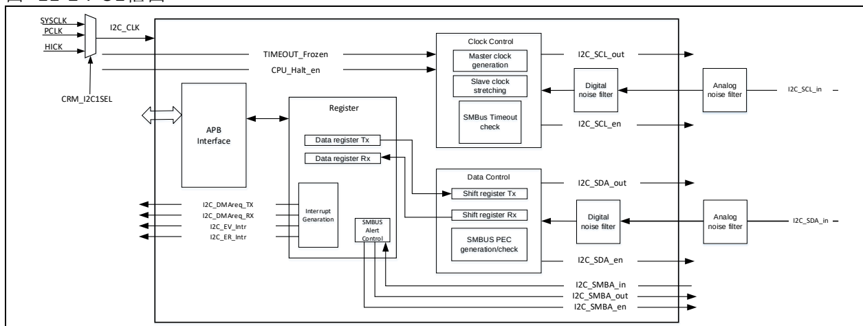
图 11-2 I 2 C1框图
