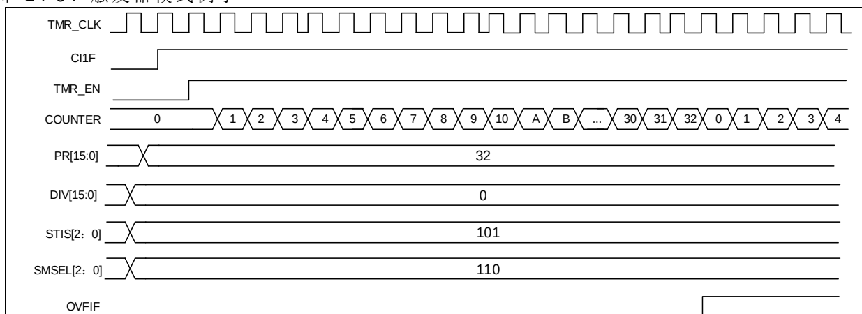
图 14-64 触发器模式例子
