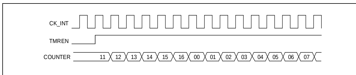
图 14-2 使用CK_INT且分频系数为1
