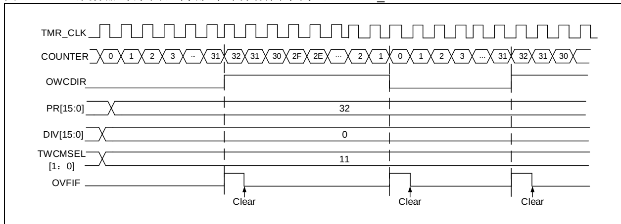
图 14-95 计数器时序图，内部时钟分频因子为0，TMRx_PR=0x32
