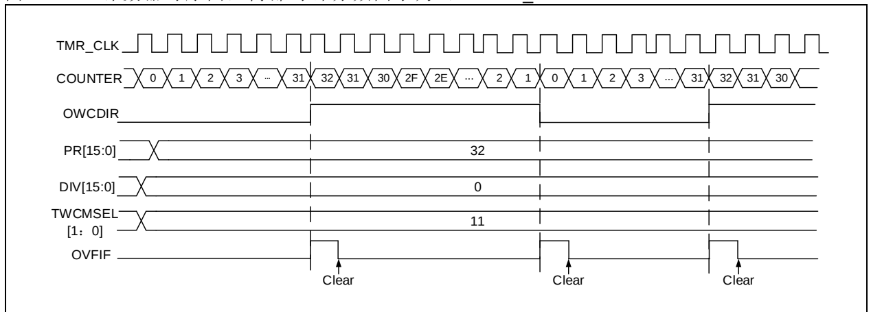
图 14-72 计数器时序图, 内部时钟分频因子为 0, TMRx_PR=0x32
