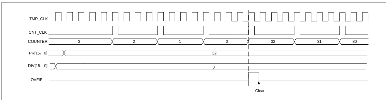
图 14-47 计数器时序图，内部时钟分频因子为3
