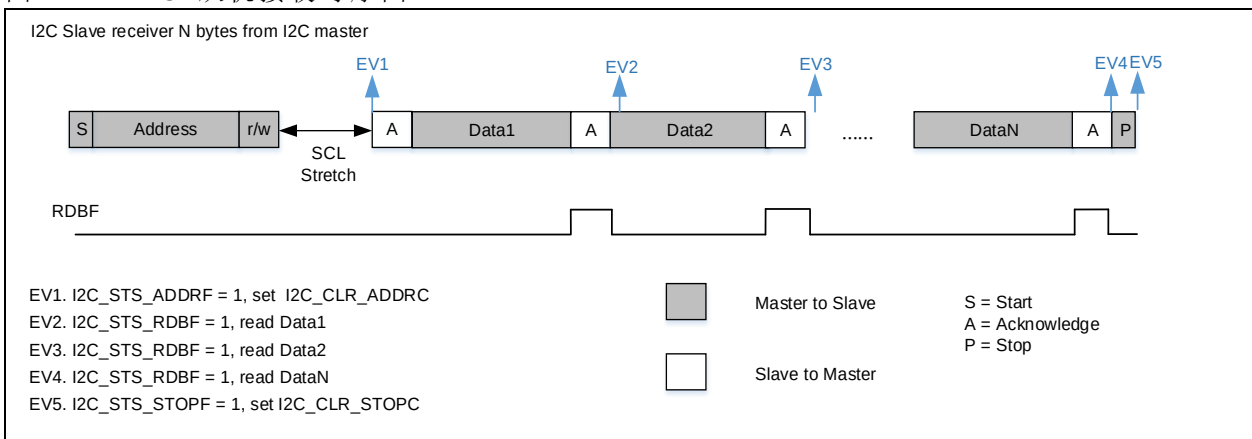
图 11-14 I 2 C 从机接收时序图
