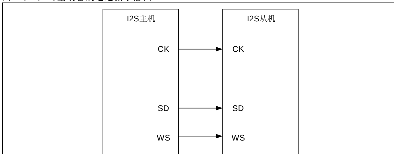
图 13-23 I 2 S主设备发送连接示意图
