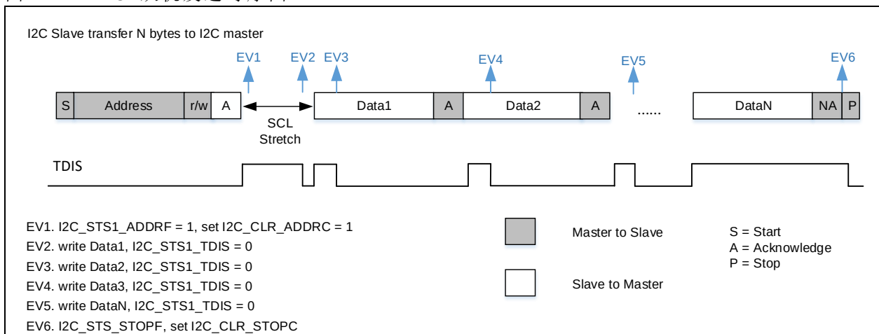
图 11-12 I 2 C 从机发送时序图
