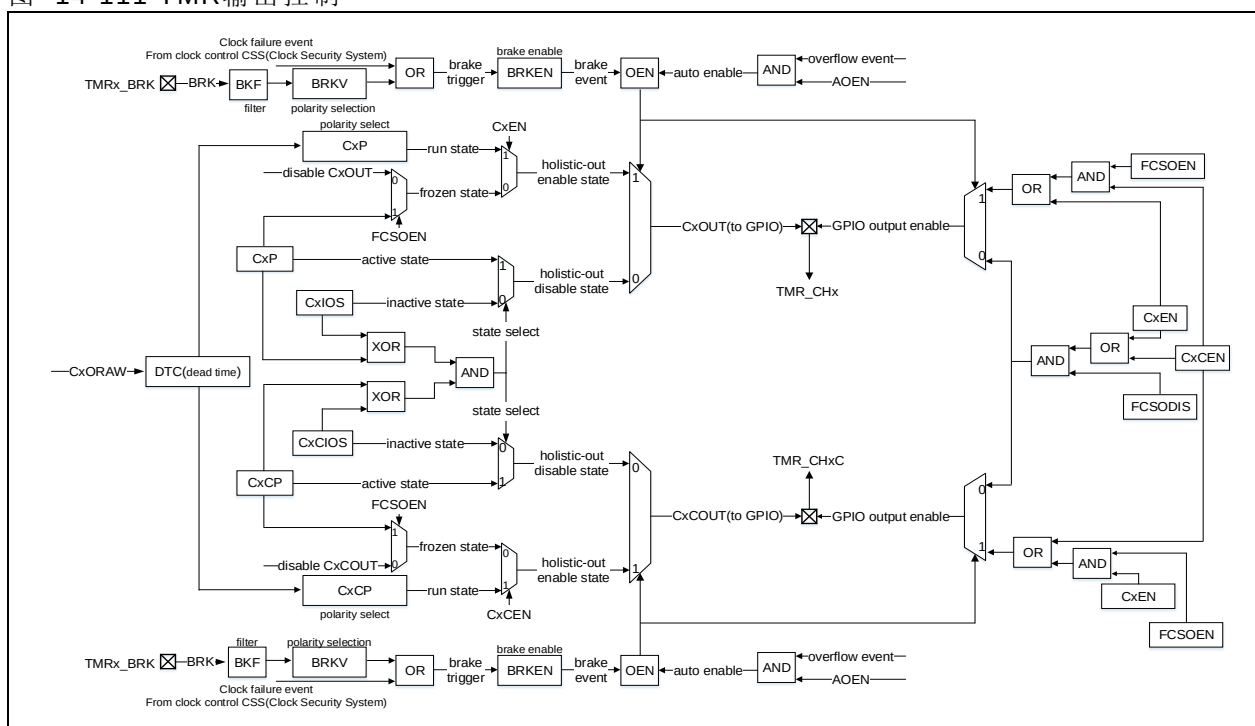
图 14-111 TMR输出控制
