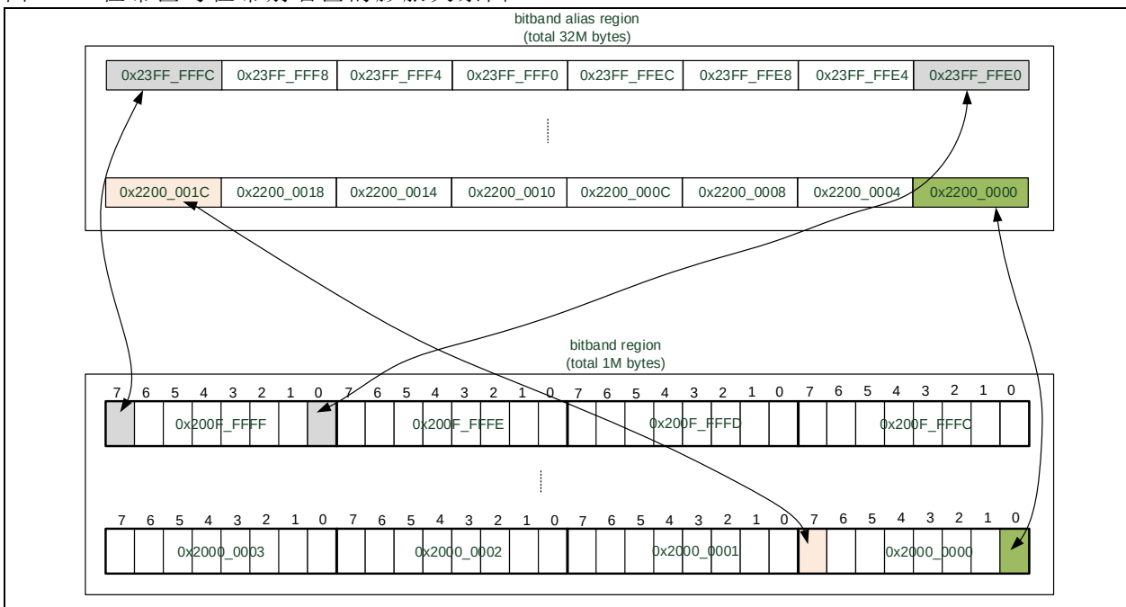
图 1-4 位带区与位带别名区的膨胀关系图B
