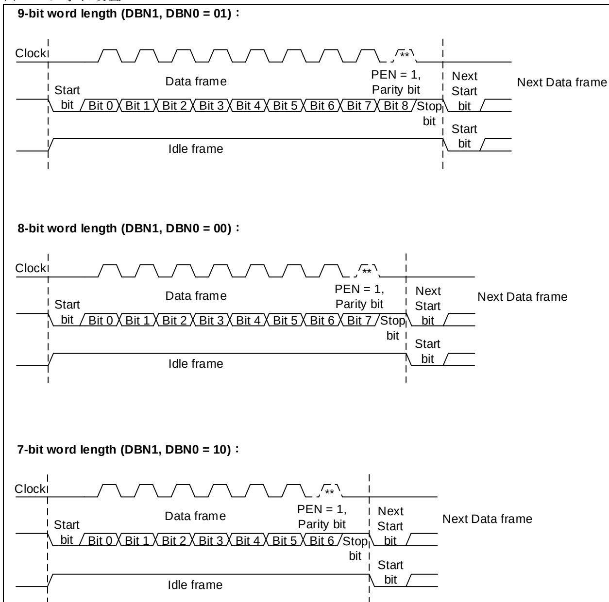
图 12-8 字长设置
