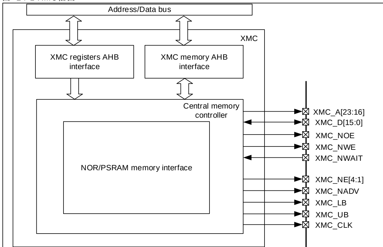
图 24-1 XMC框图
