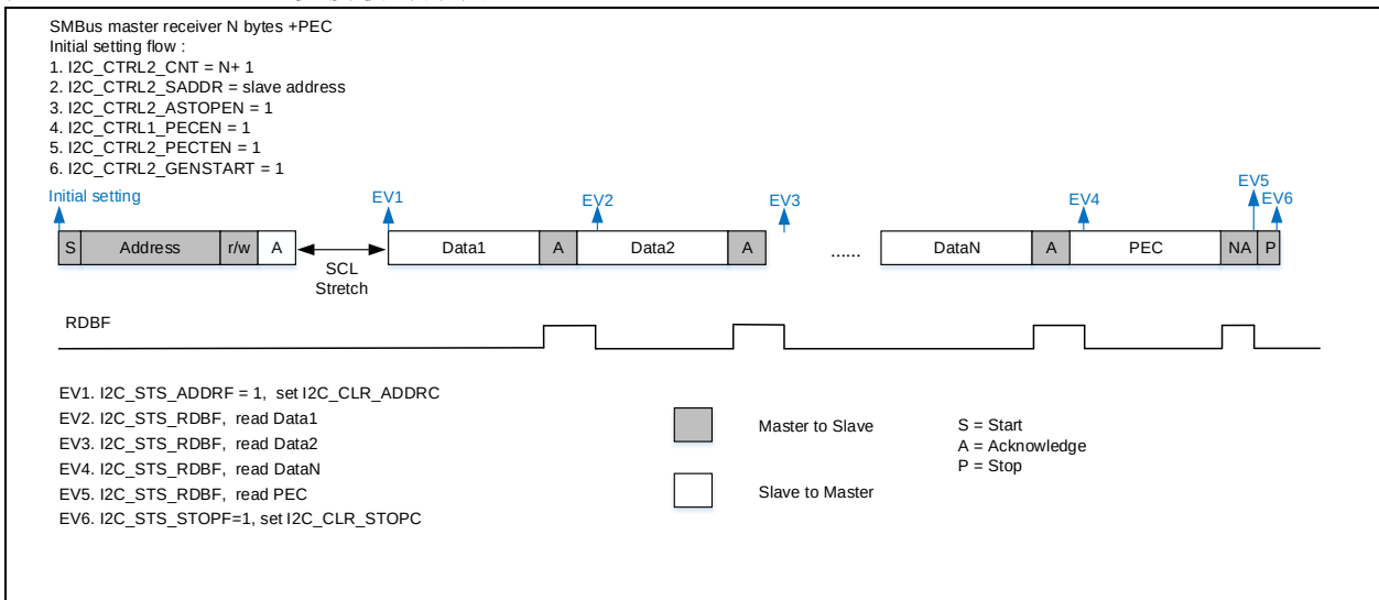
图 11-18 SMBus主机接收时序图
