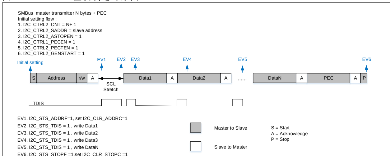
图 11-16 SMBus主机发送时序图
