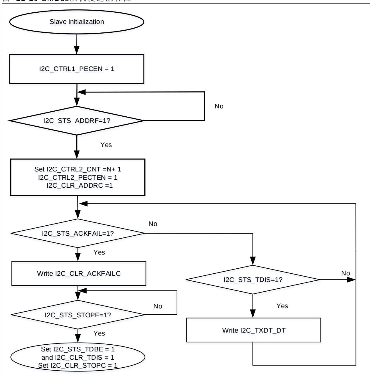
图 11-19 SMBus从机发送流程图
