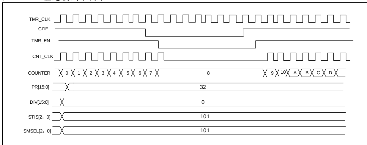
图 14-114 挂起模式下例子
