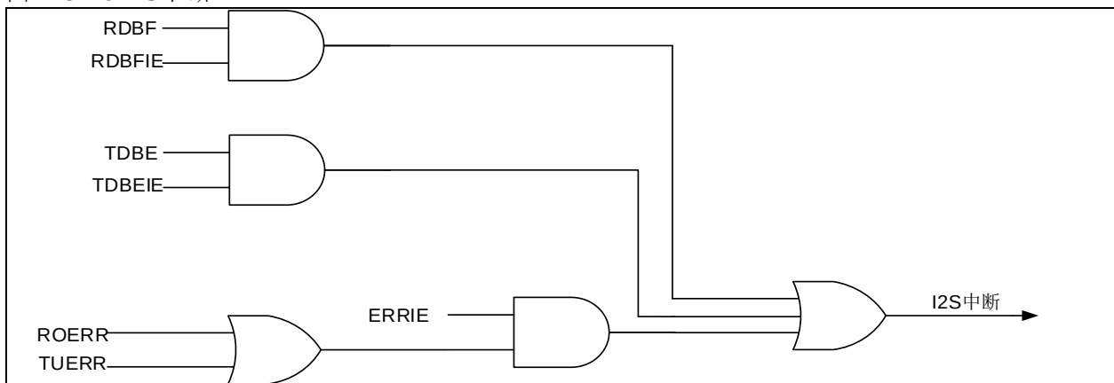
图 13-26 I 2 S中断
