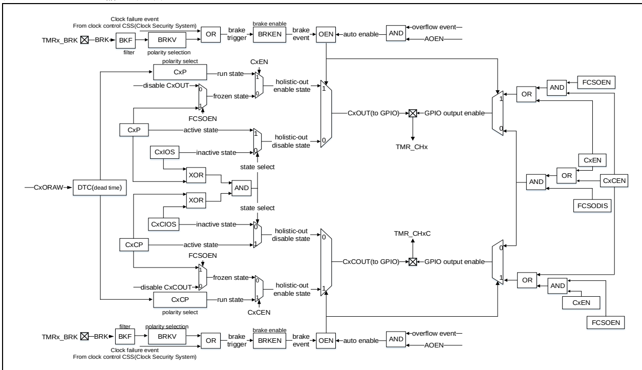
图 14-60 TMR 输出控制
