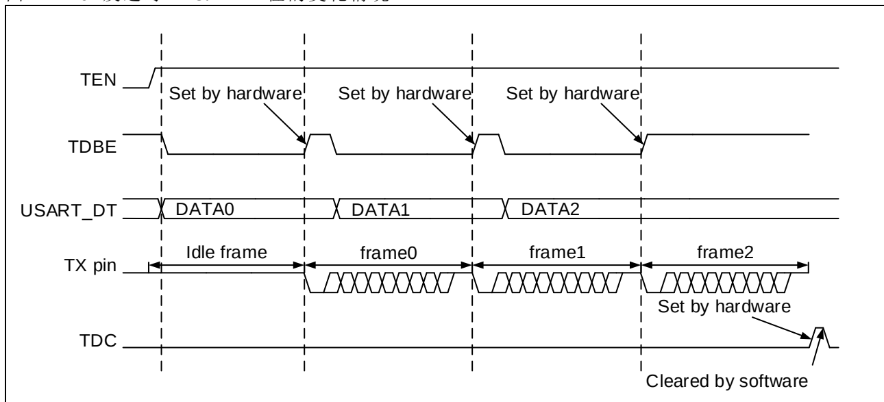
图 12-10 发送时 TDC/TDBE 位的变化情况
