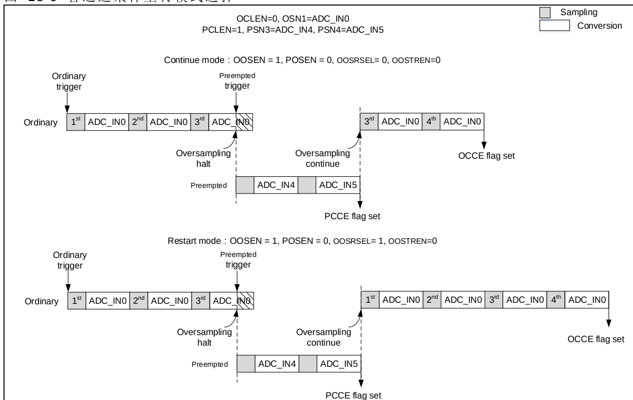
图 18-9 普通过采样重转模式选择
