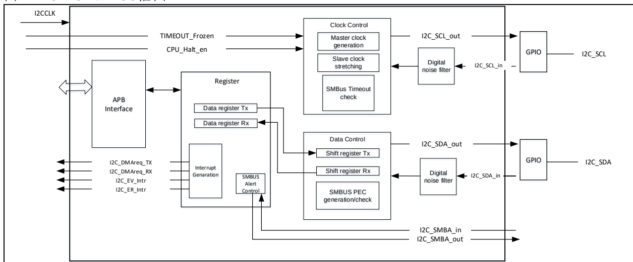
图 11-3 I 2 C2、I 2 C3框图
