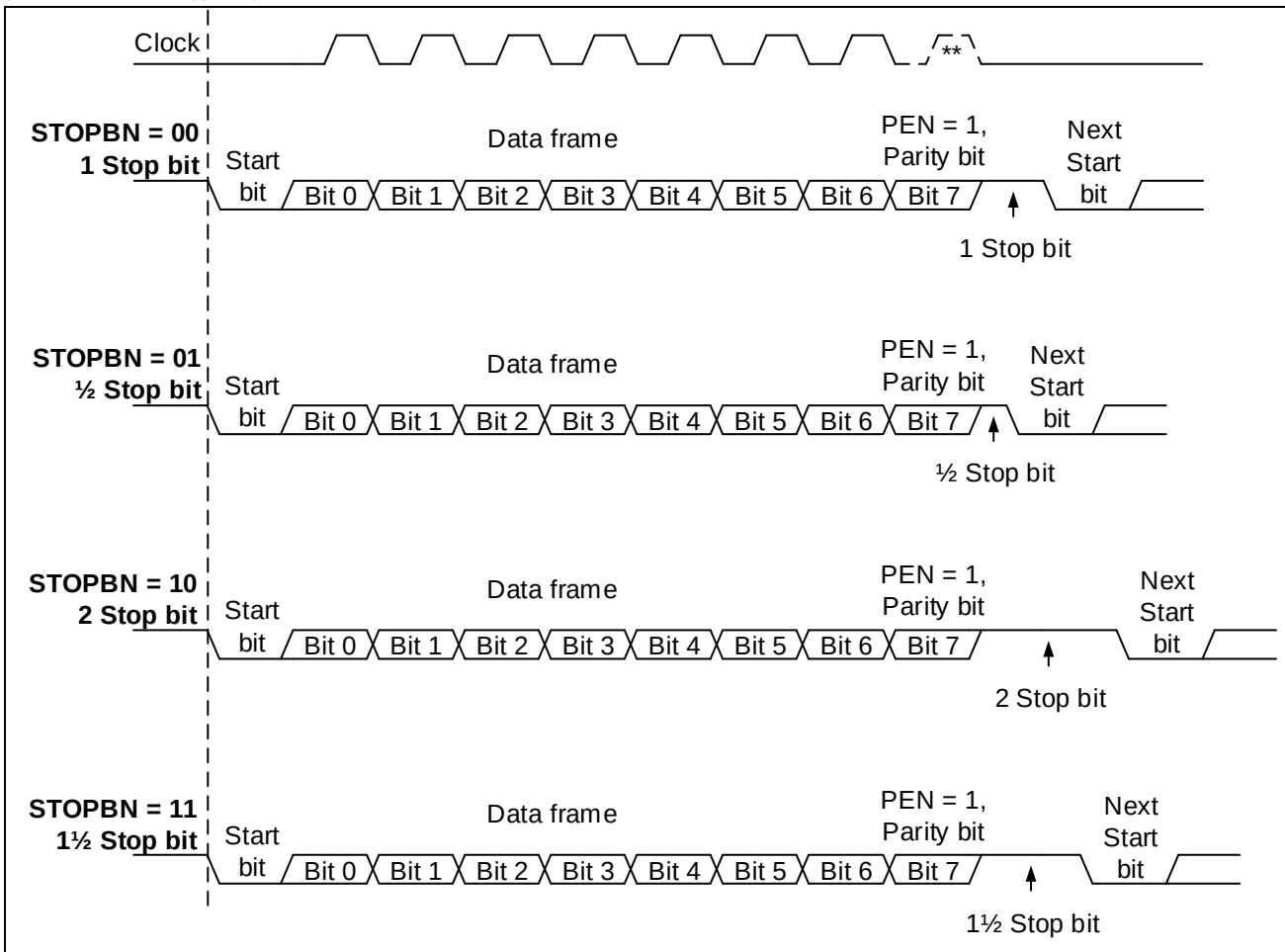
图 12-9 配置停止位
