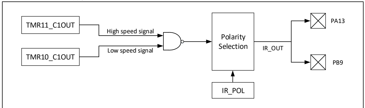
图 23-1 IRTMR结构框图
