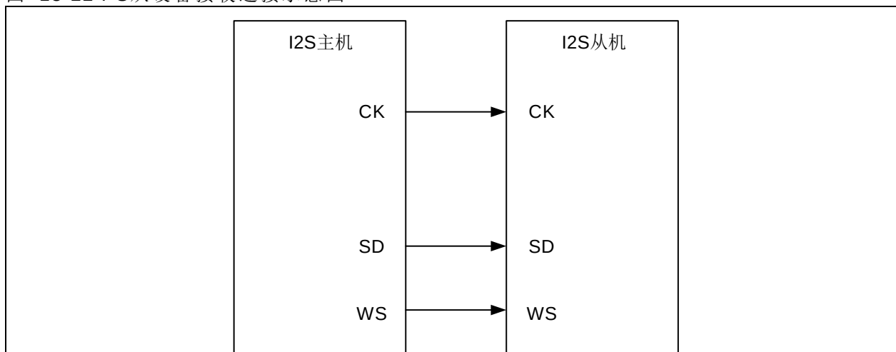
图 13-22 I 2 S从设备接收连接示意图
