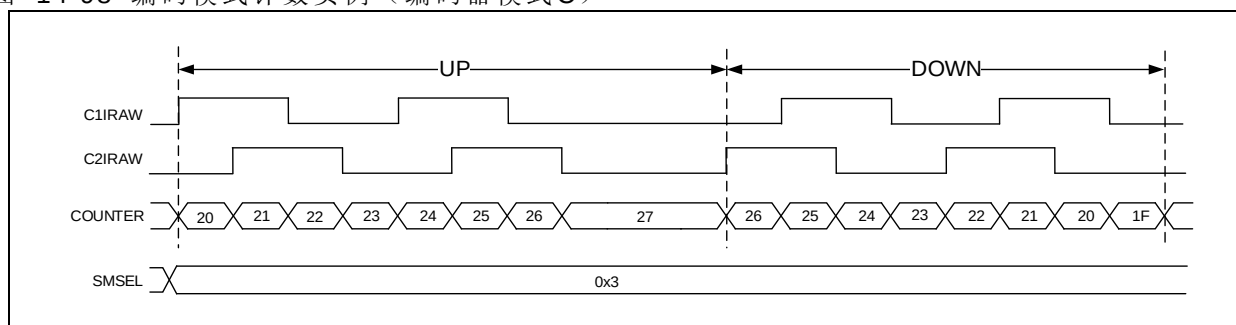
图 14-98 编码模式计数实例 (编码器模式 C)
