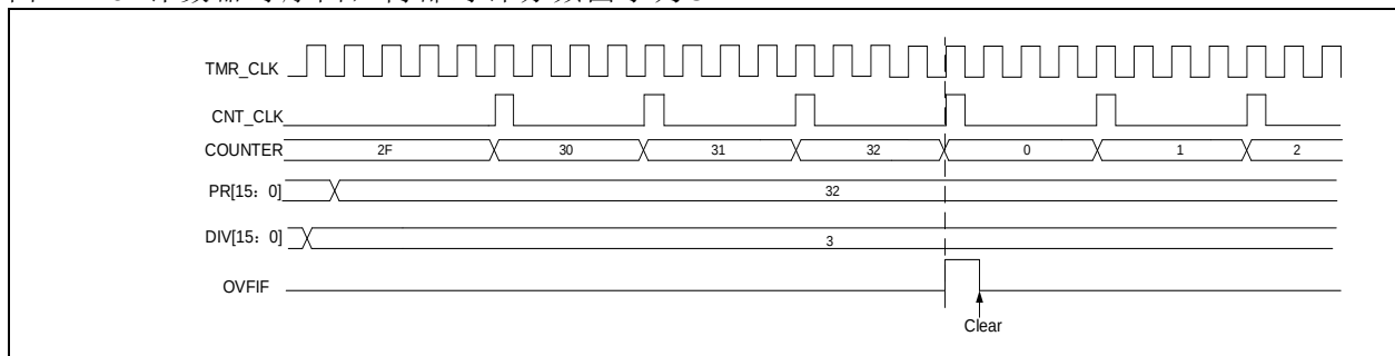
图 14-6 计数器时序图，内部时钟分频因子为3
