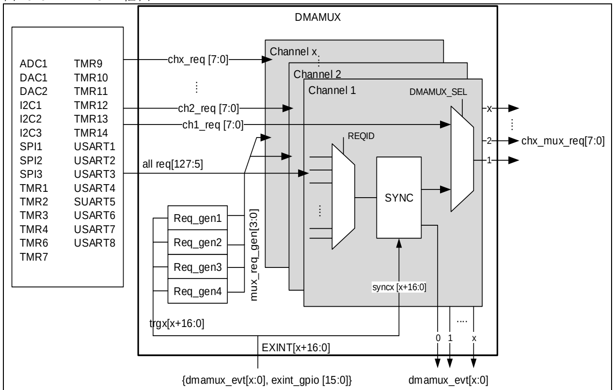
图 9-6 DMAMUX 框图
