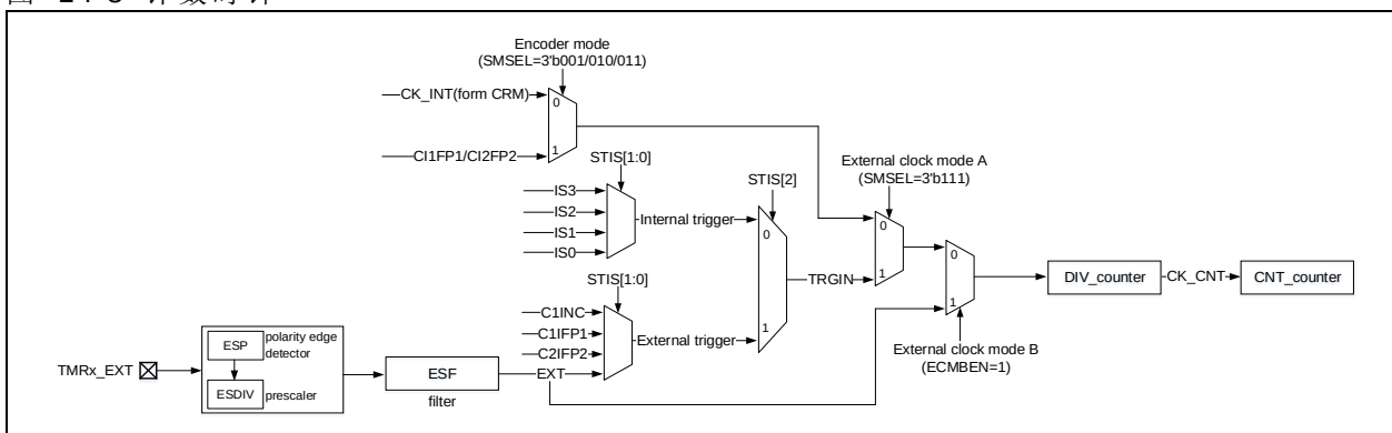
图 14-8 计数时钟
