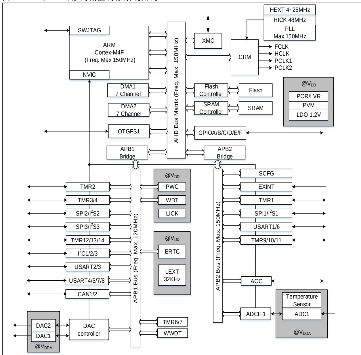
图 1-1 AT32F423系列微控制器系统架构
