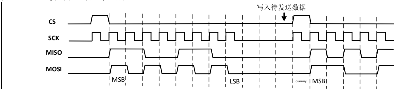
图 13-16 TI模式非连续通信时序
