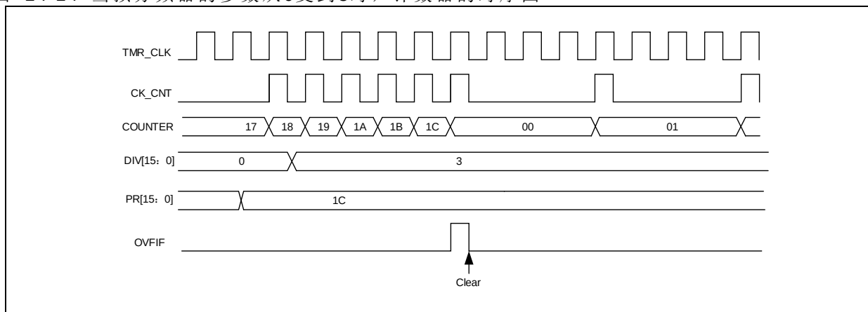
图 14-14 当预分频器的参数从0变到3时，计数器的时序图
