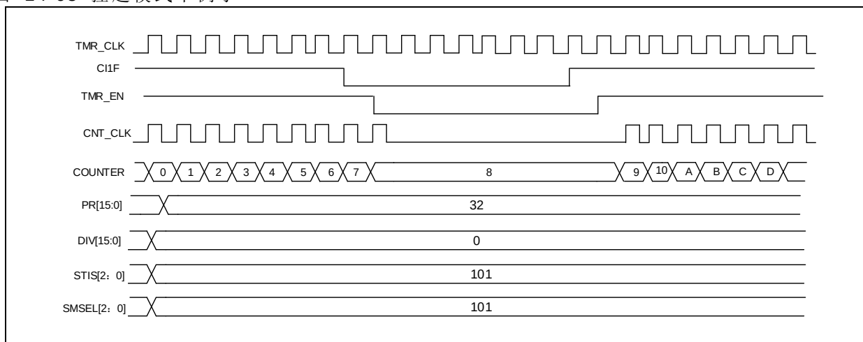
图 14-63 挂起模式下例子
