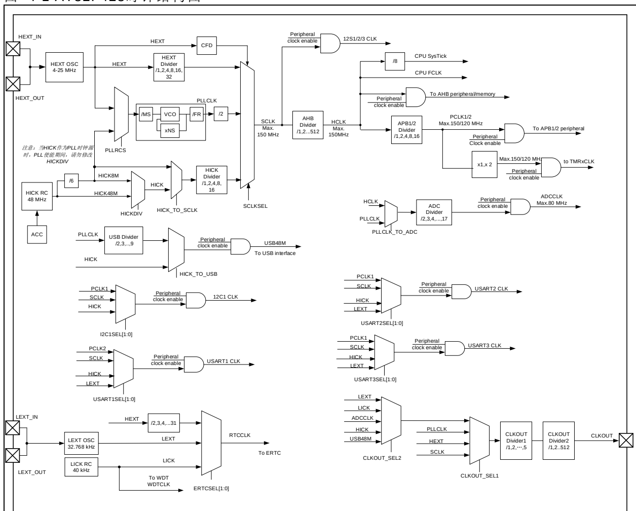
图 4-1 AT32F423时钟结构图
