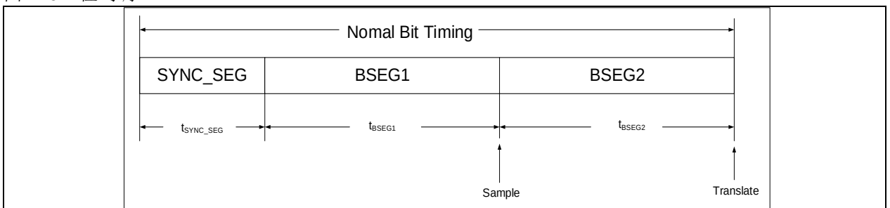
图 20-1 位时序
