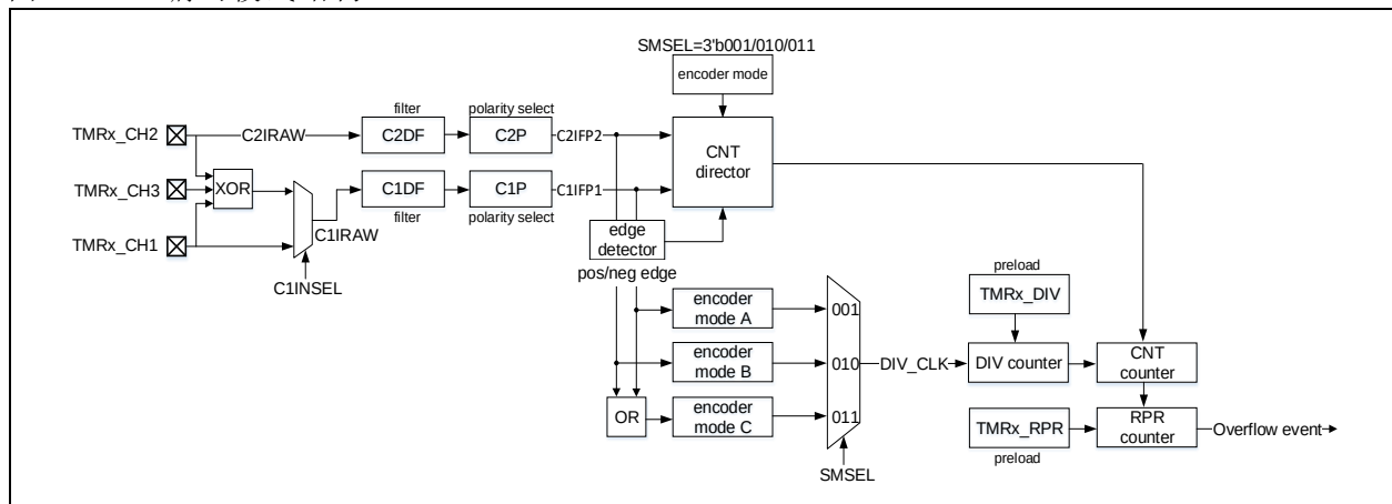
图 14-97 编码模式结构
