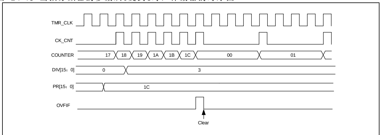
图 14-43 当预分频器的参数从0变到3时，计数器的时序图
