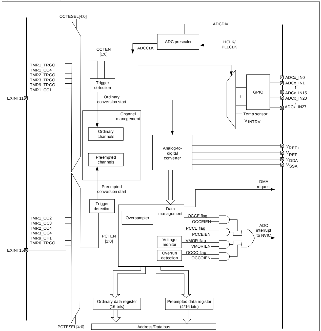
图 18-1 ADC1框图
