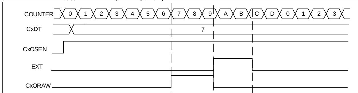
图 14-109 EXT清除CxORAW(PWM模式B)
