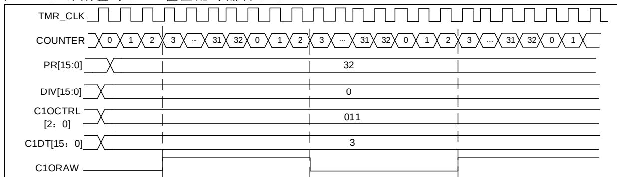
图 14-78 计数值与C1DT值匹配时翻转C1ORAW
