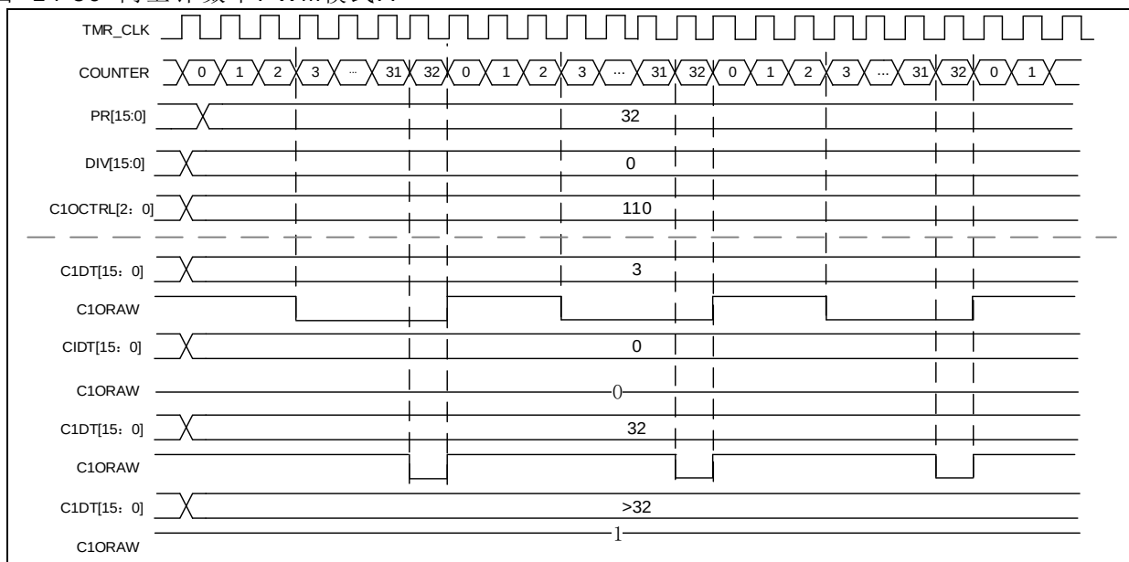
图 14-56 向上计数下 PWM 模式 A
