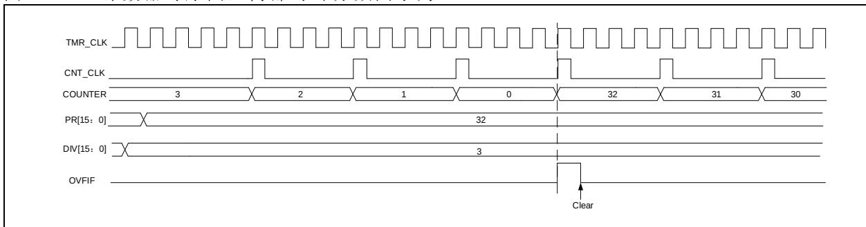
图 14-94 计数器时序图，内部时钟分频因子为 3
