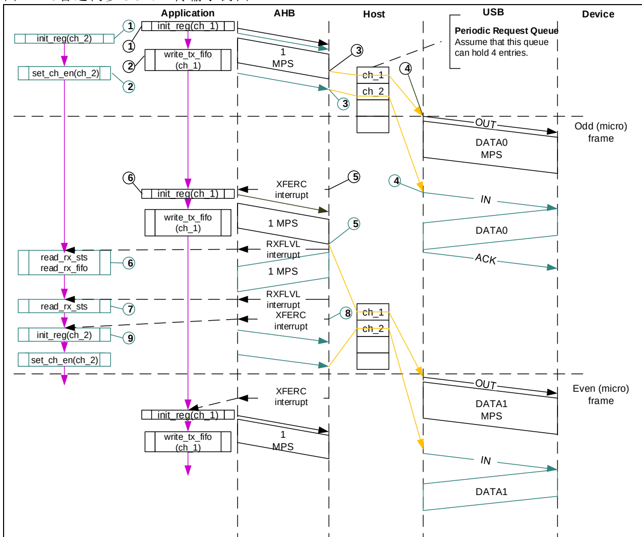
图 21-9普通同步OUT/IN传输示例图
