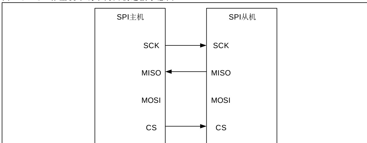
图 13-4 SPI 作主机单线单向只收连接示意图
