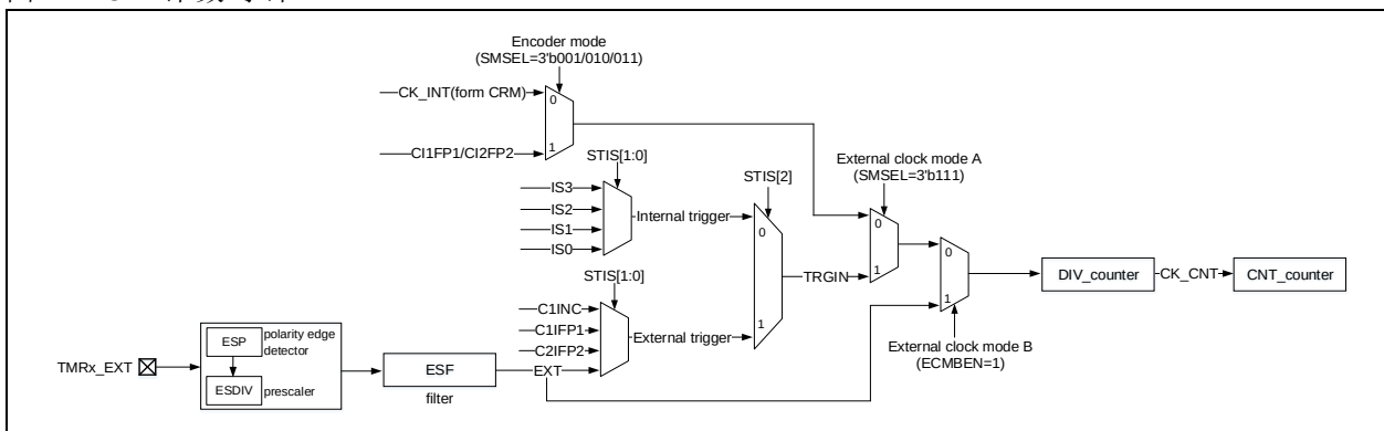
图 14-84 计数时钟
