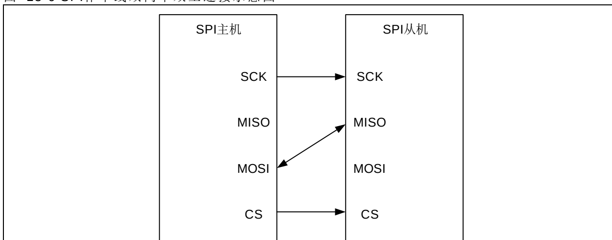
图 13-6 SPI作单线双向半双工连接示意图
