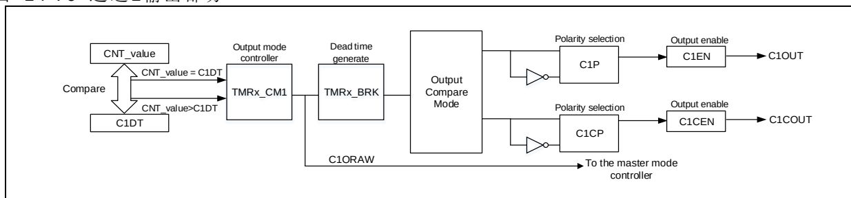
图 14-76 通道1输出部分
