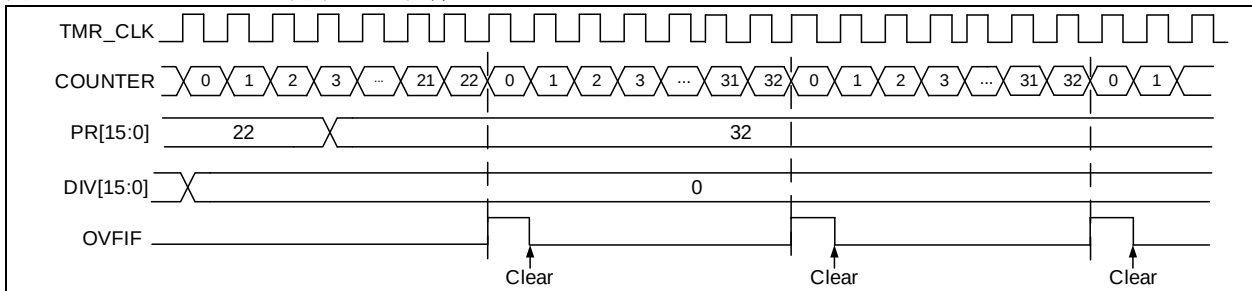
图 14-46 PRBEN=1时的溢出事件
