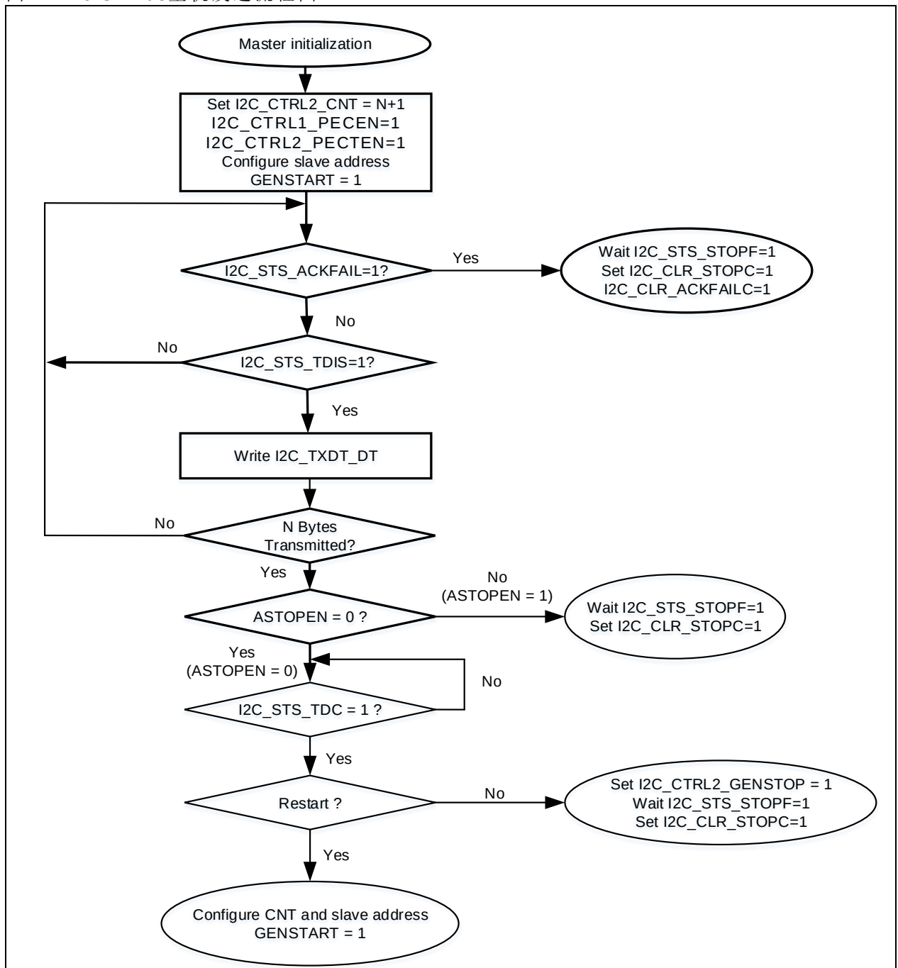
图 11-15 SMBus主机发送流程图
