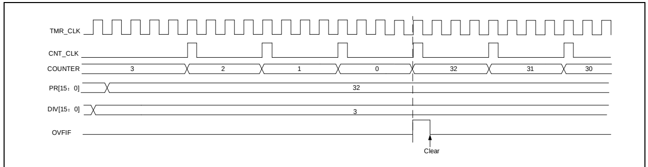
图 14-71 计数器时序图, 内部时钟分频因子为 3
