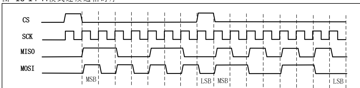
图 13-14 TI模式连续通信时序
