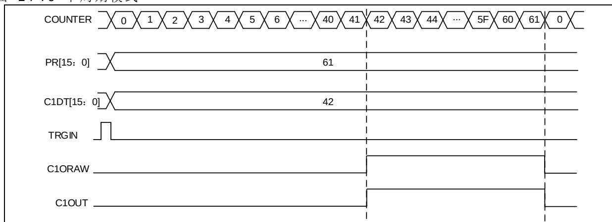
图 14-79 单周期模式
