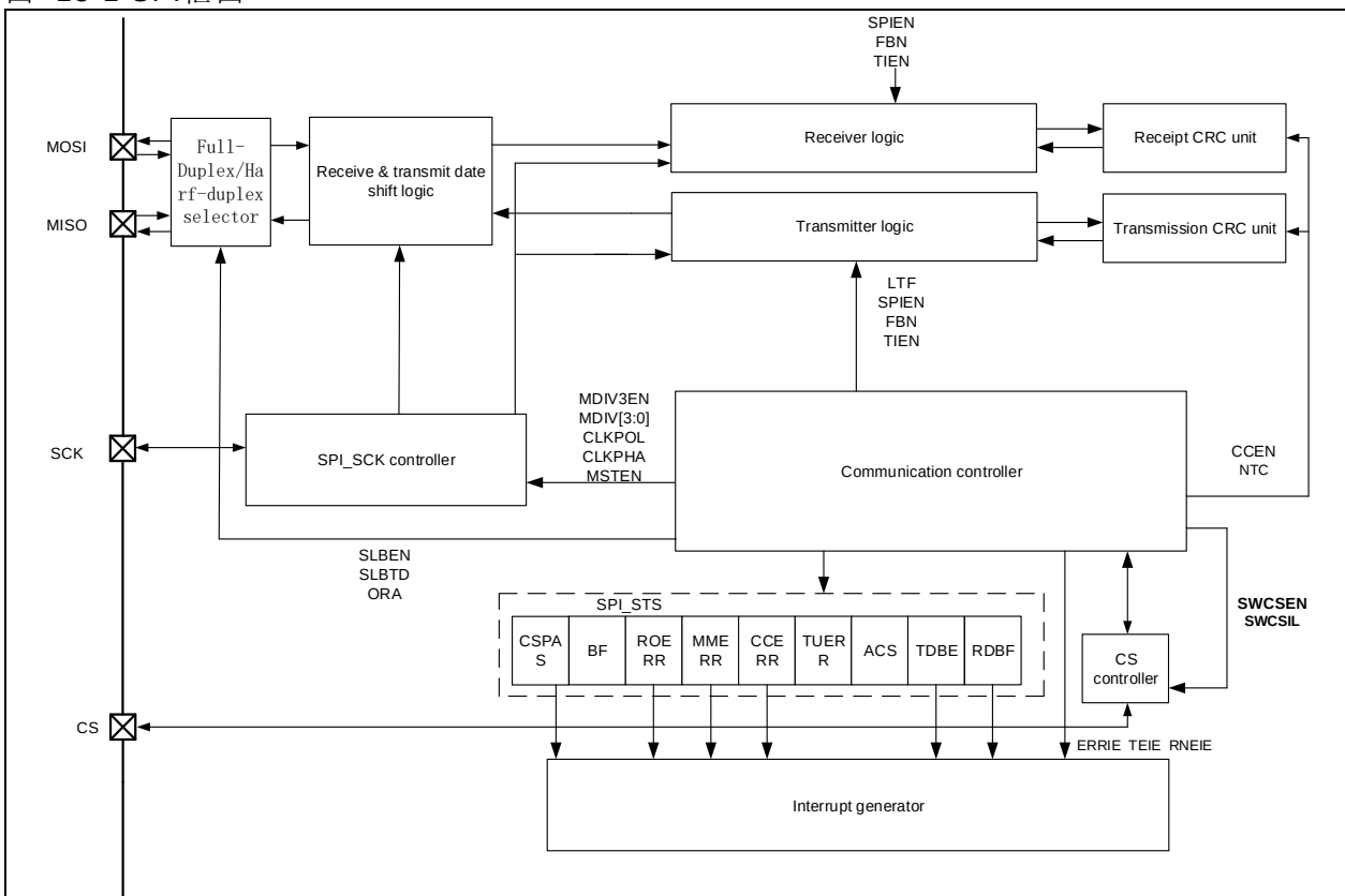
图 13-1 SPI框图
