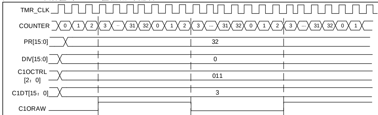
图 14-57 计数值与 C1DT 值匹配时翻转 C1ORAW
