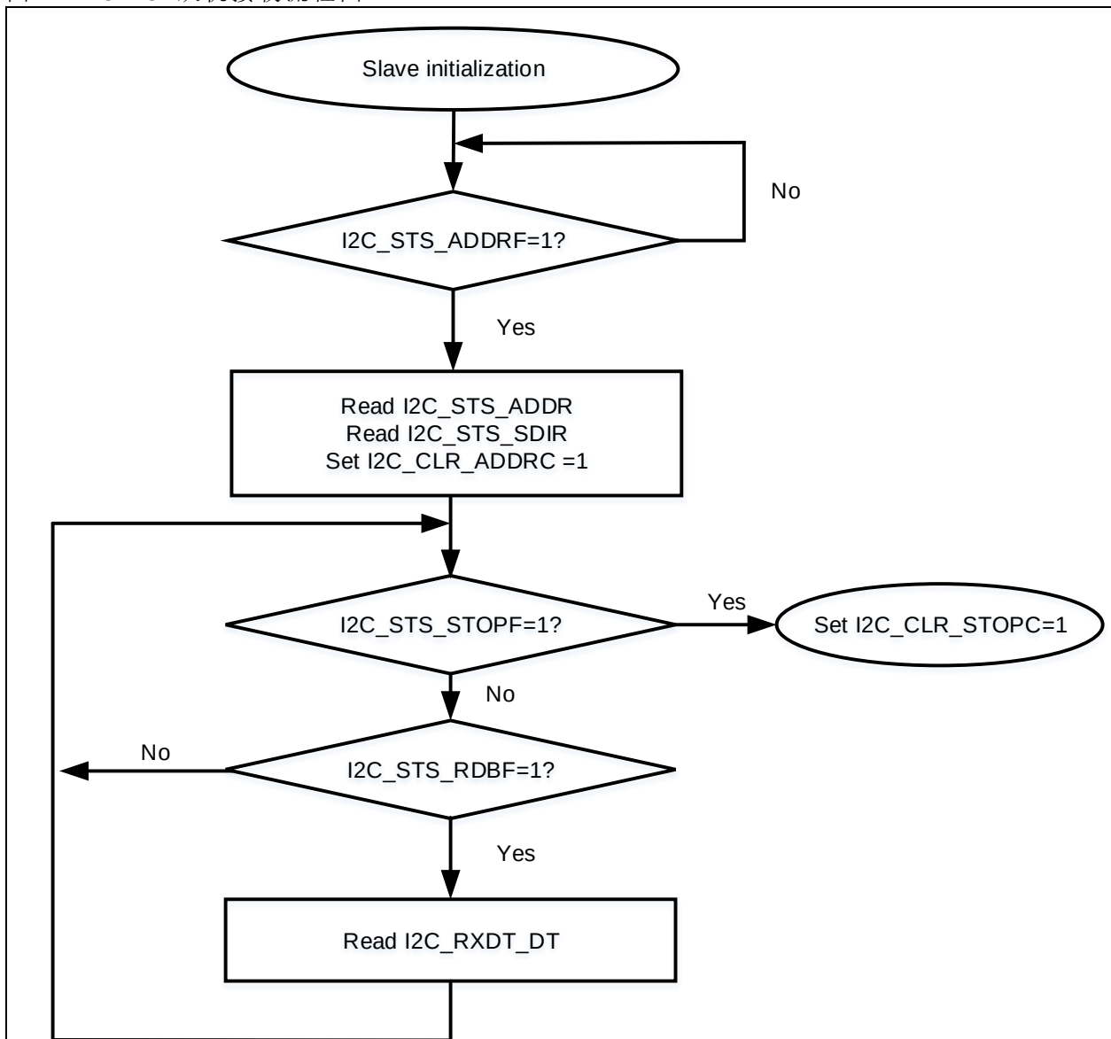
图 11-13 I 2 C 从机接收流程图
