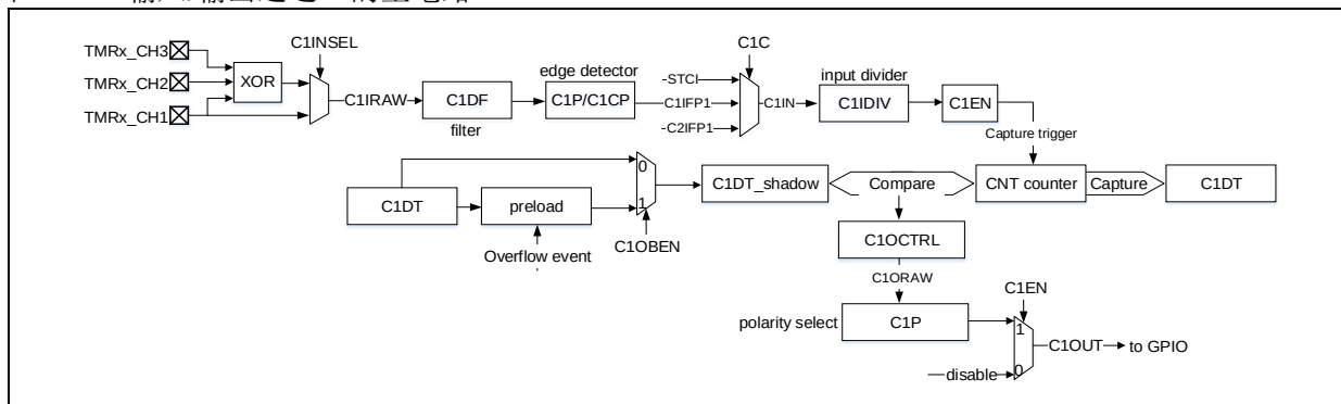
图 14-23 通道 1 输入部分
