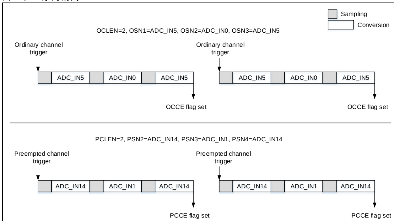
图 18-4 序列模式
