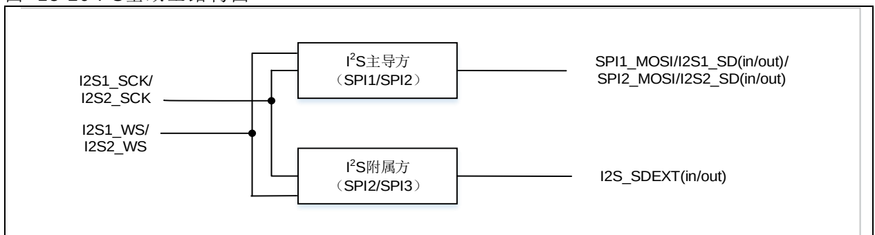
图 13-20 I 2 S全双工结构图
