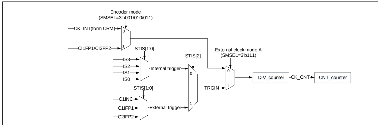
图 14-39 计数时钟
