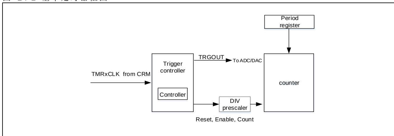
图 14-1 基本定时器框图
