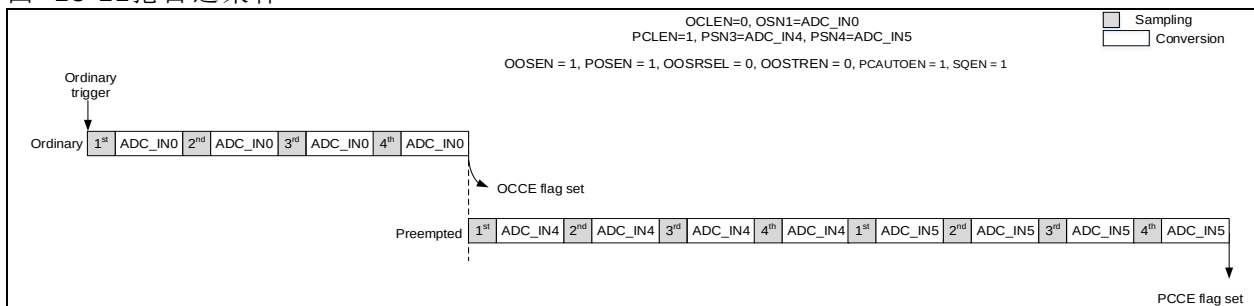
图 18-11 抢占过采样
