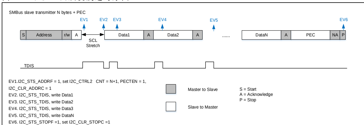
图 11-20 SMBus从机发送时序图
