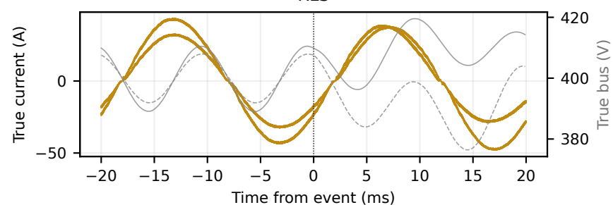
H (v5)
