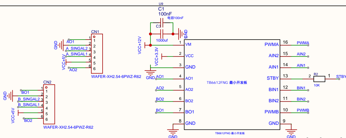
电机电路
