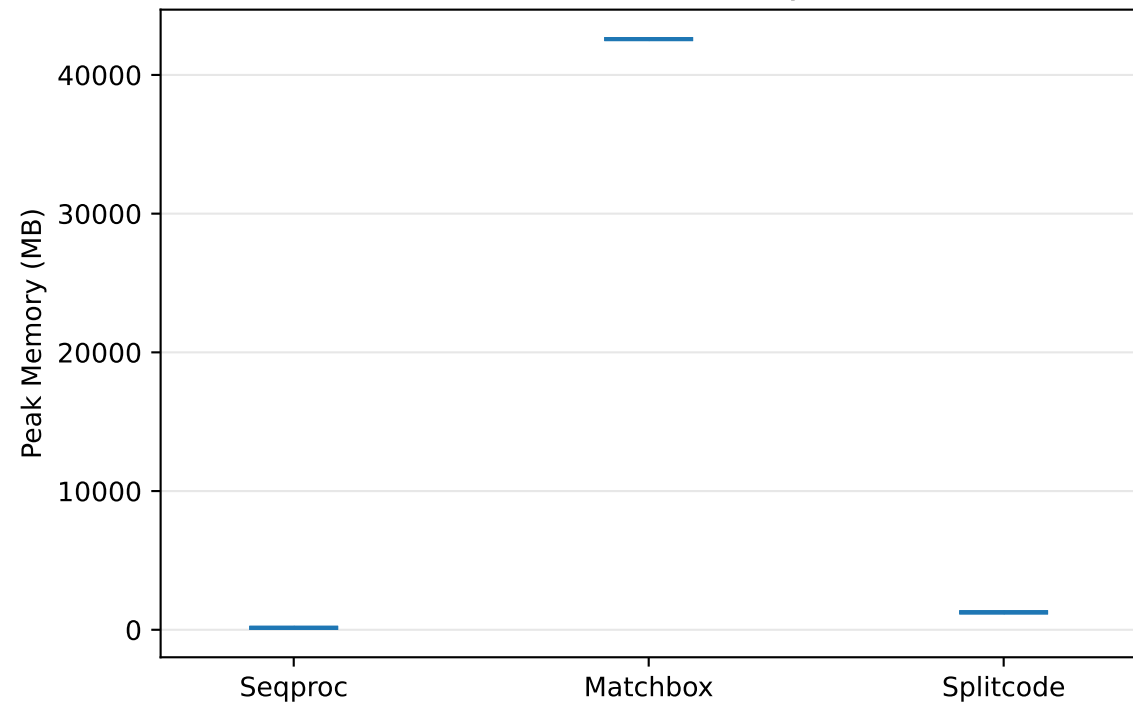
sci-RNA-seq3 - Memory
