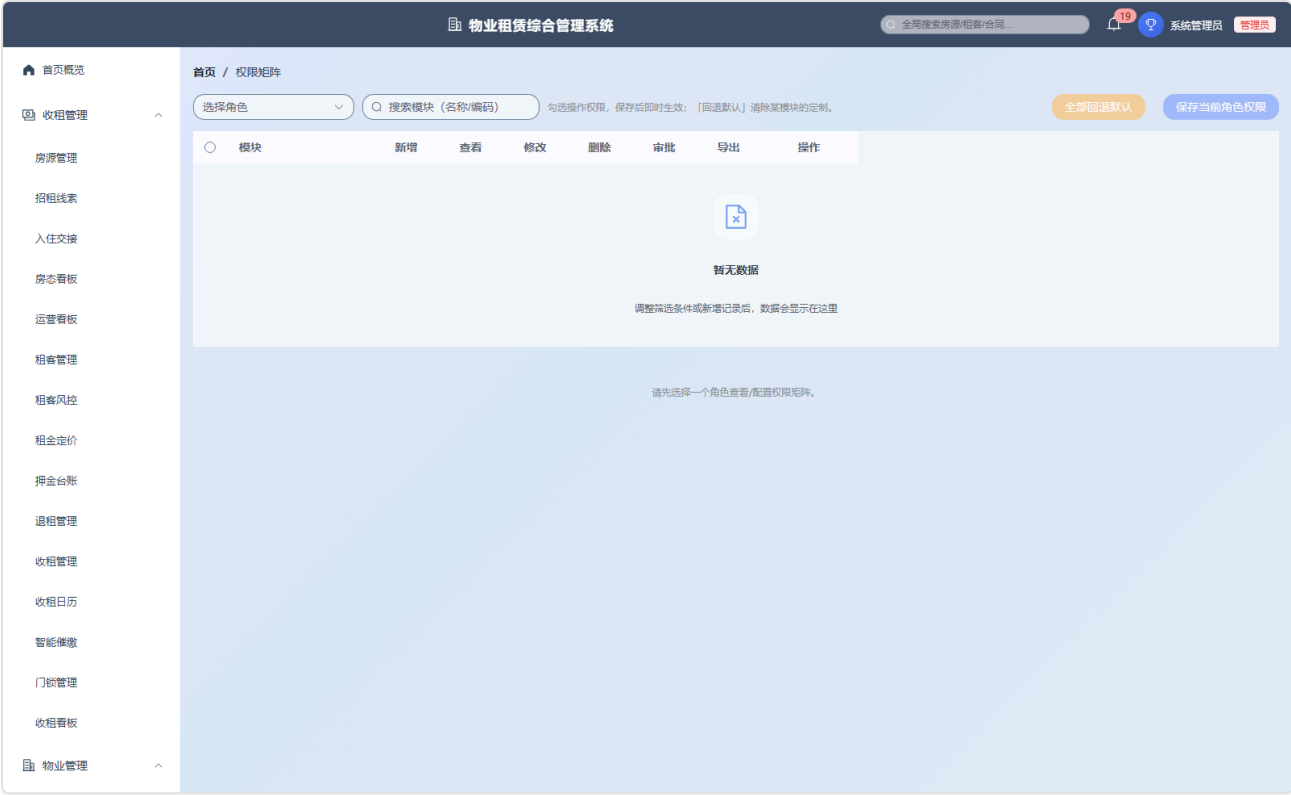
权限矩阵
