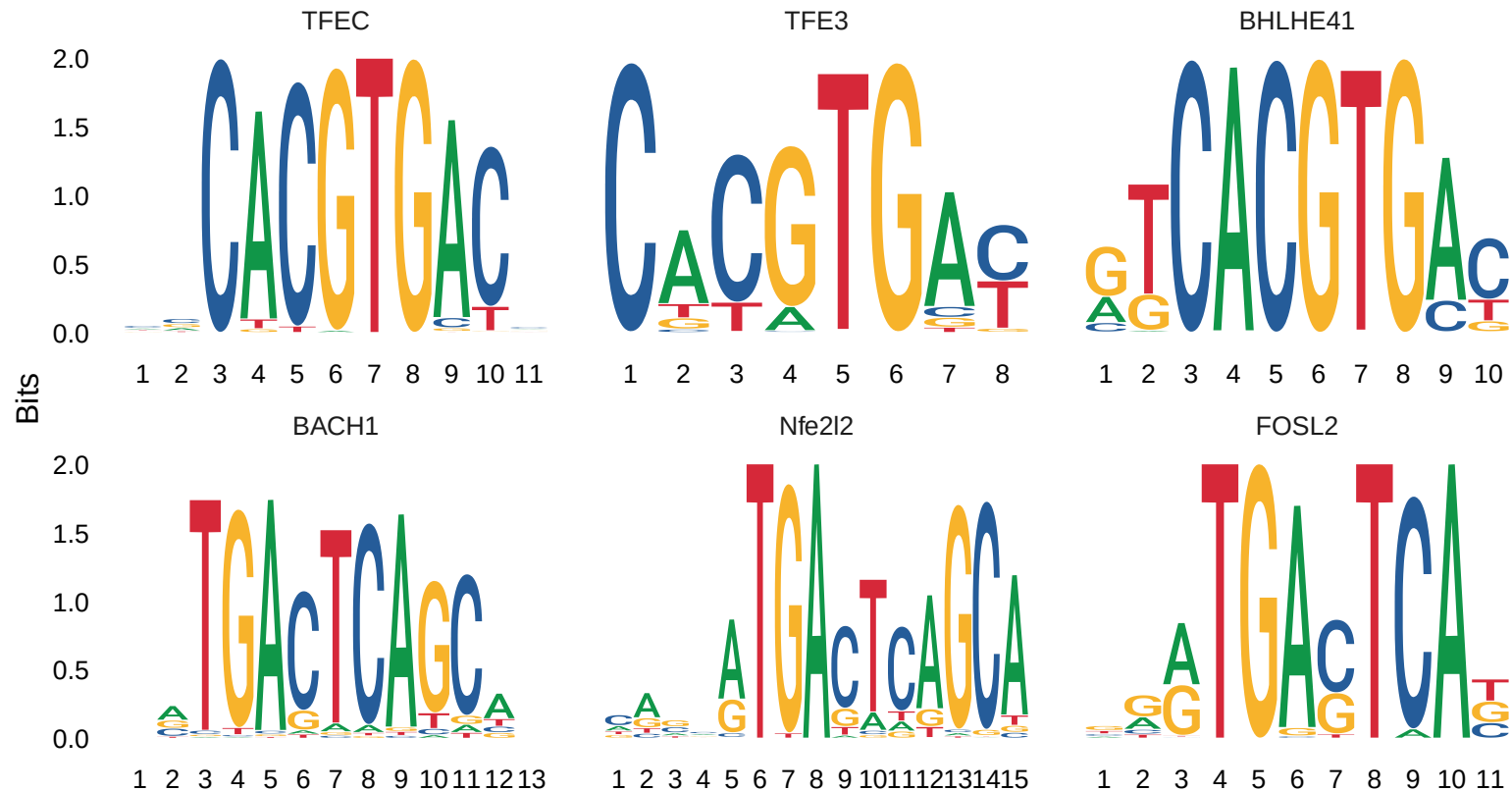
Fig. 4I motif logos
