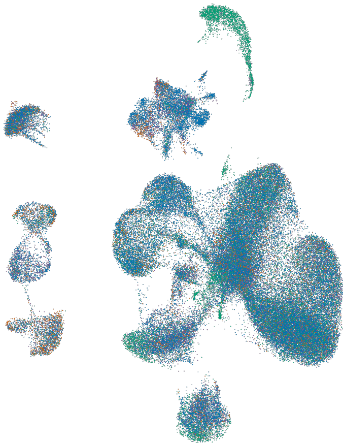
diffuse30
