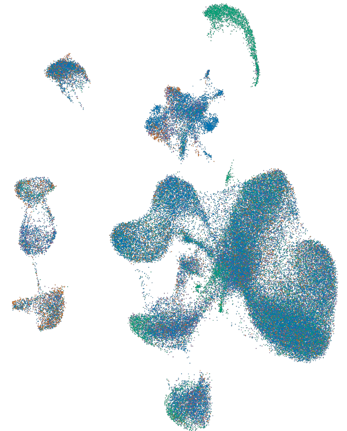
diffuse50
