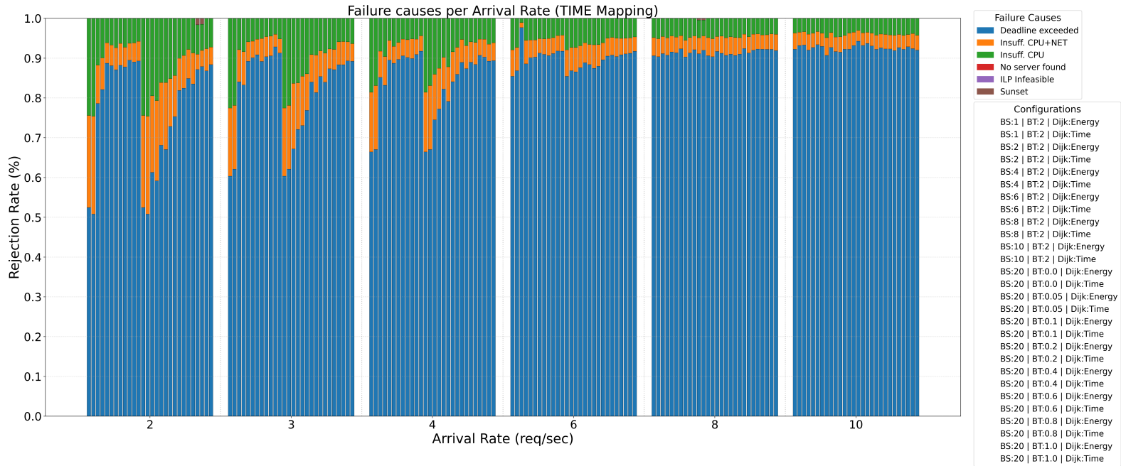
Figura 5: Distribuzione delle Cause di Rigetto sul totale dei task (Configurazione Time).
