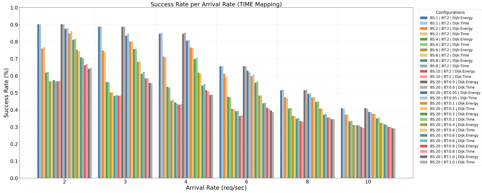
Figura 4: Success Rate - Configurazione Time.
