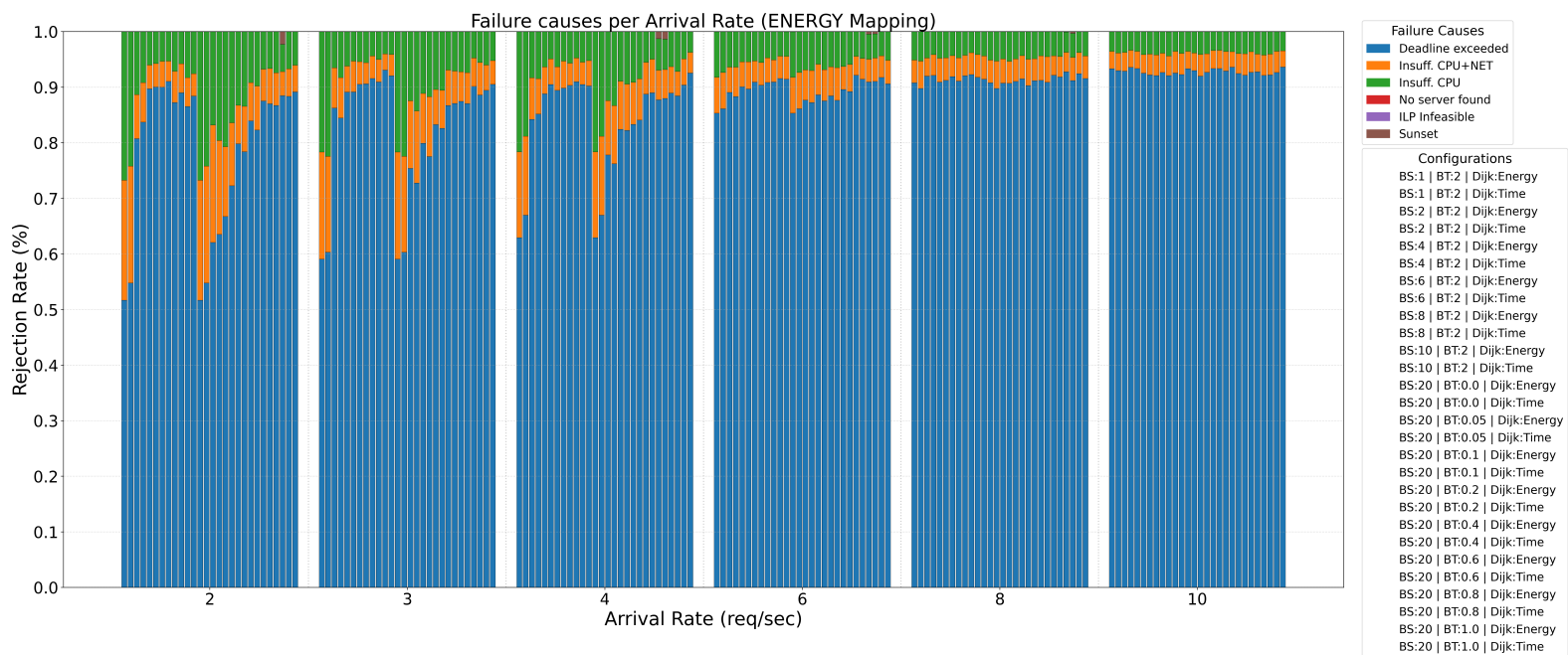
Figura 2: Distribuzione delle Cause di Rigetto sul totale dei task (Configurazione Energy).
