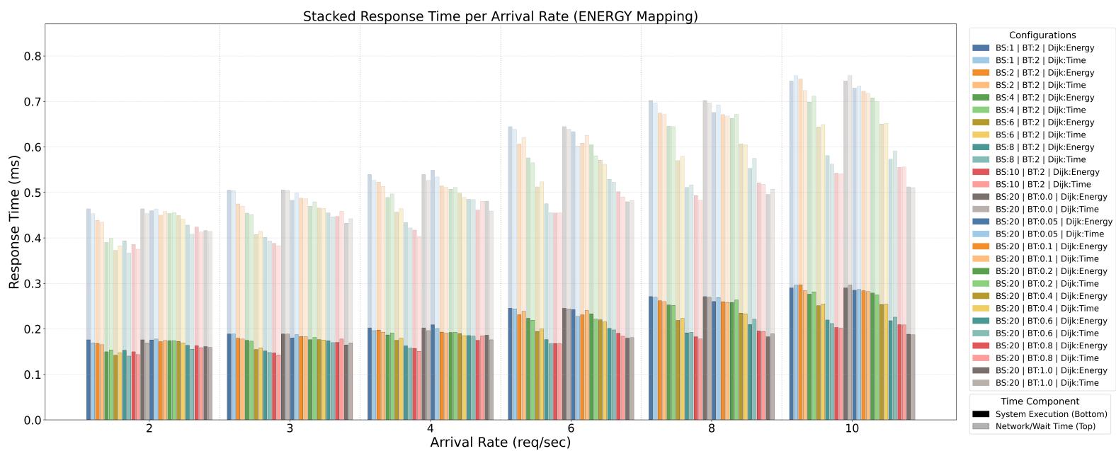
Figura 3: Scomposizione del Response Time (Configurazione Energy).
