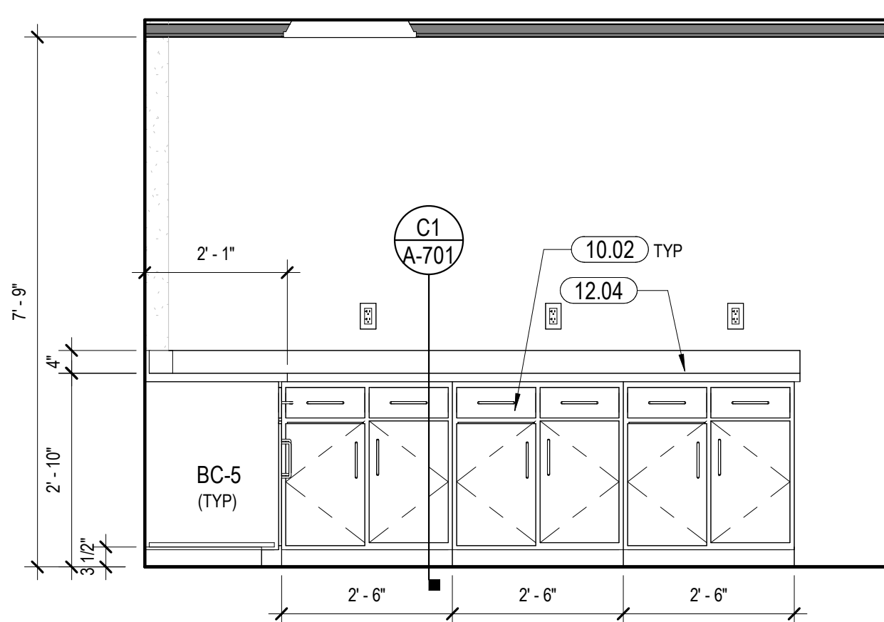
E9 LOUNGE/CAFE - INT EL 1 1/2" = 1'-0"
