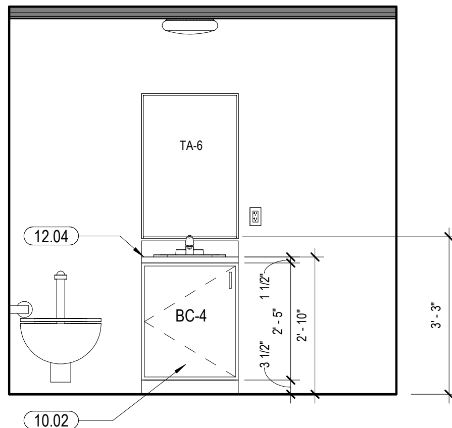
(K9) BATHROOM - RM 103 - INT EL 3 1/2" = 1'-0"
