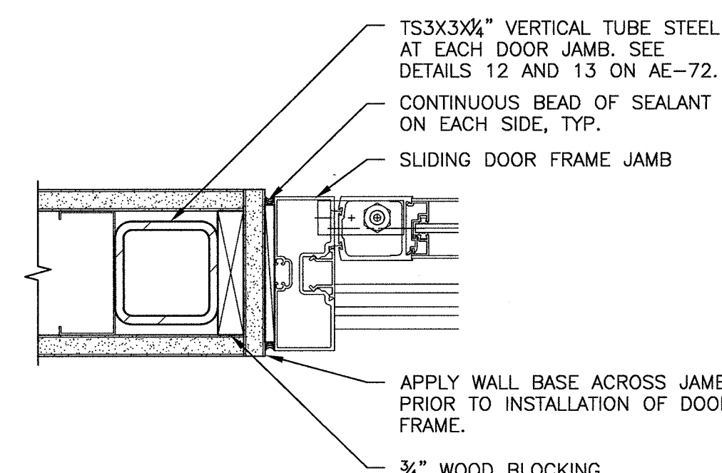
7 SLIDING DOOR JAMB DETAIL
