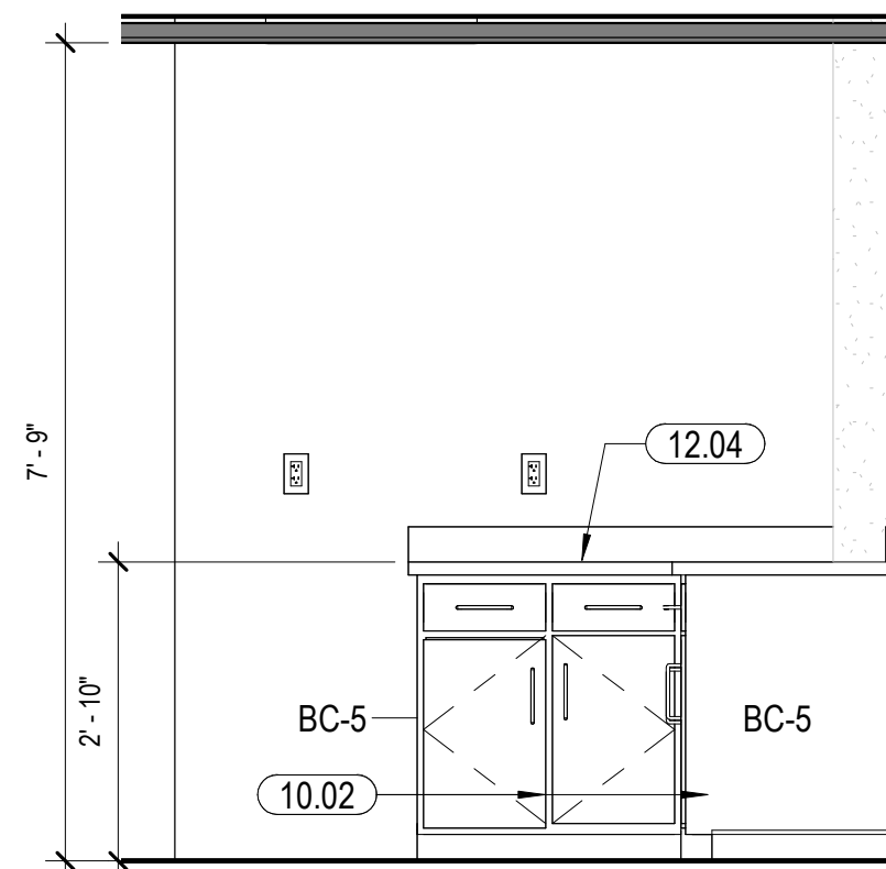
E13 LOUNGE/CAFE - INT EL 2 1/2" = 1'-0"
