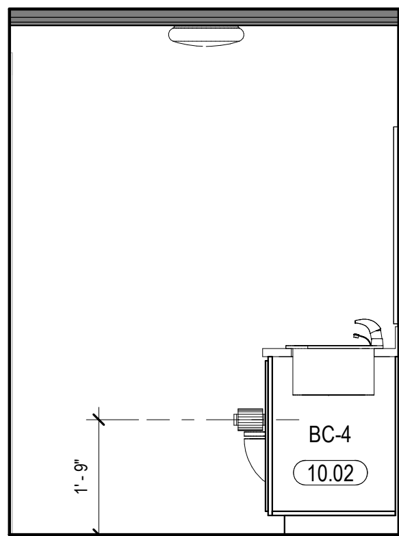
(K5) BATHROOM - RM 103 - INT EL 2 1/2" = 1'-0"
