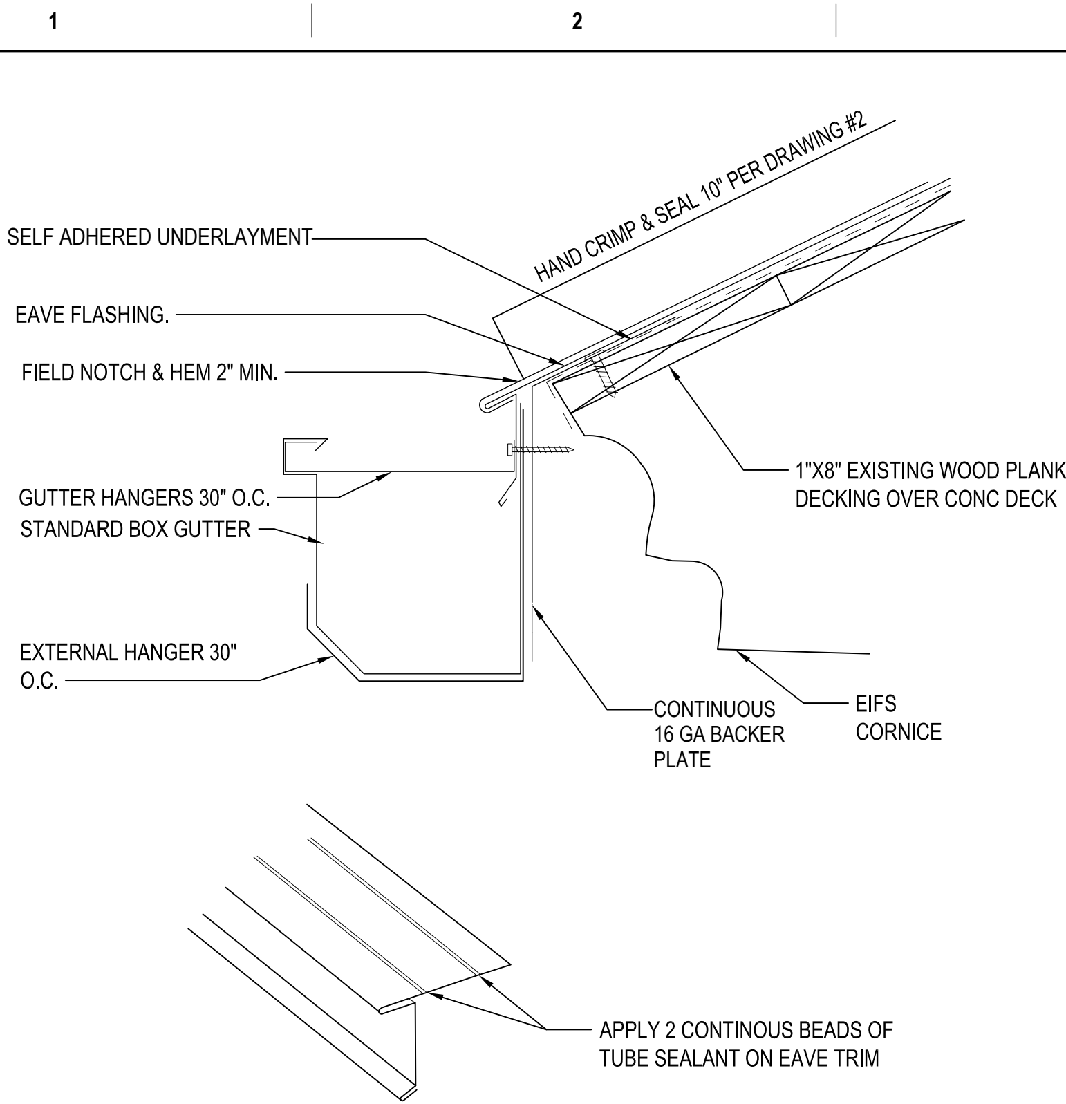
1 GUTTER DETAIL AE503 SCALE: 1-1/2"=1'-0"
