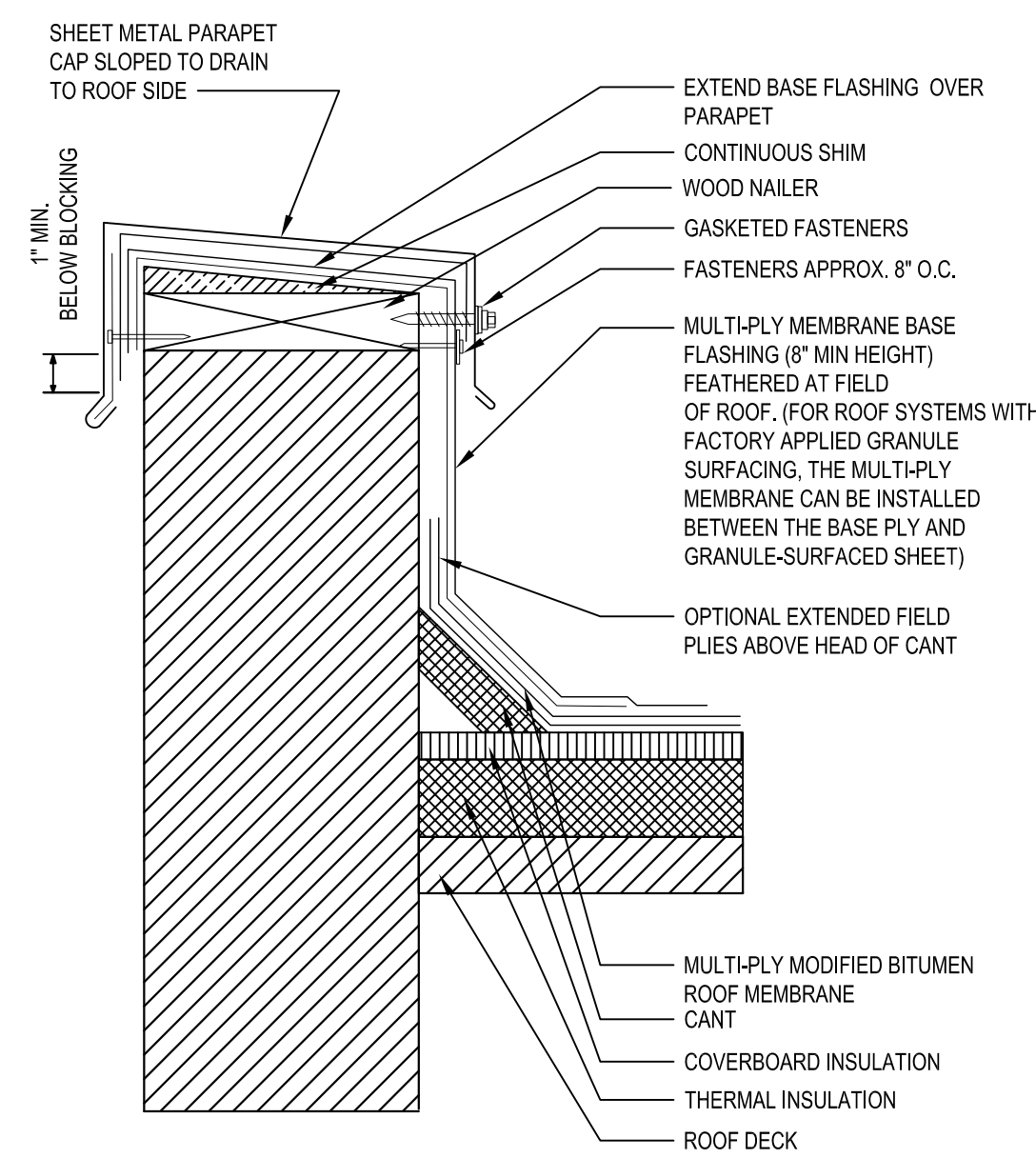
11 PARAPET CAP DETAIL AE503 SCALE: 1-1/2"=1'-0"
