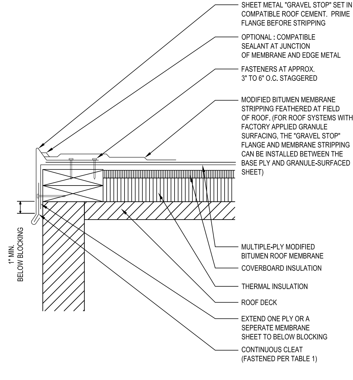
10 EDGE GUARD DETAIL AE503 SCALE: 1-1/2"=1'-0"
