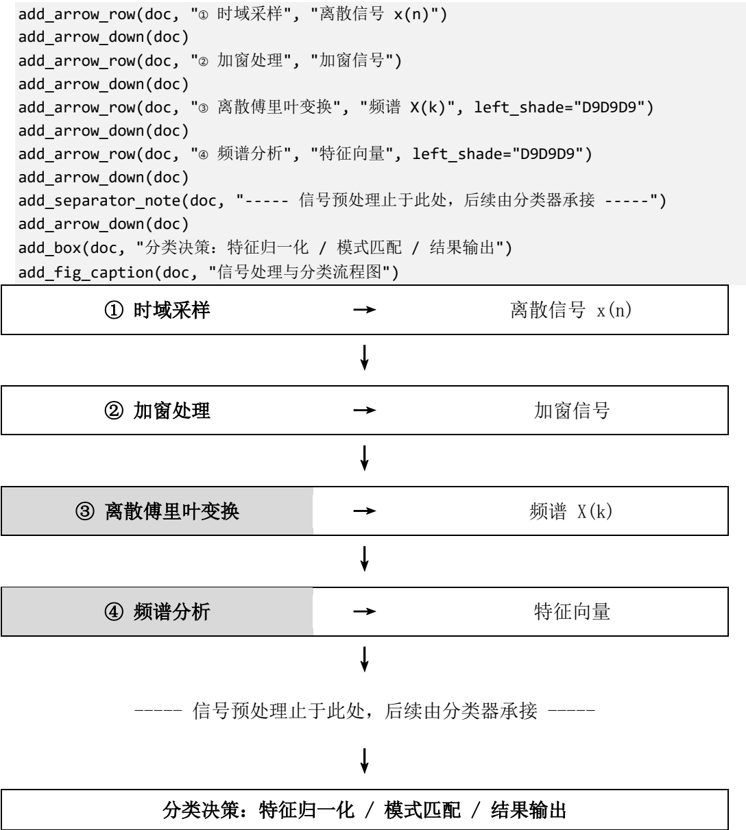
图 2 信号处理与分类流程图
