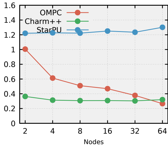
(d) FFT
