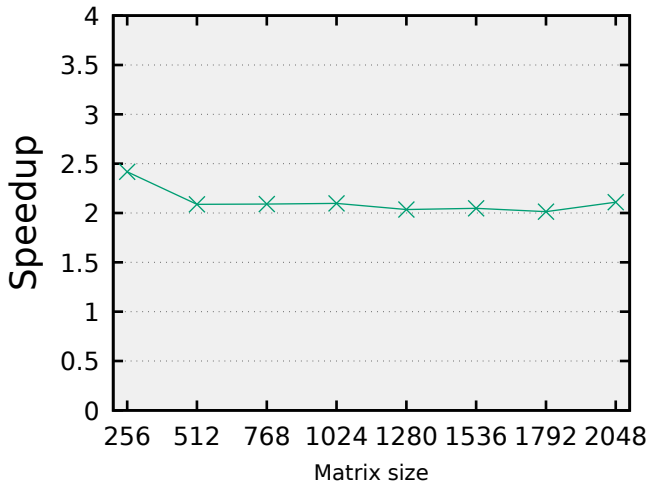
(b) SGEMV
