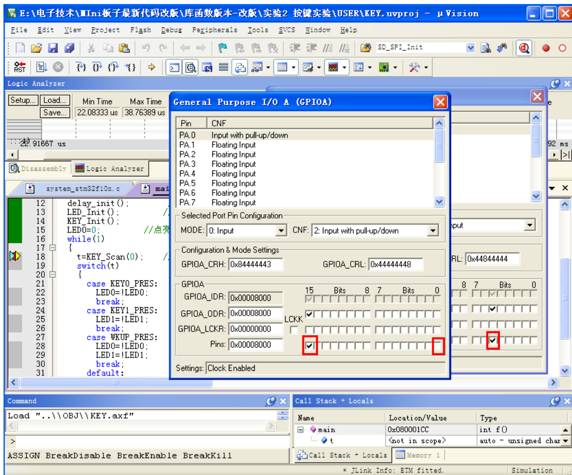
图 7.4.3 执行到断点处
