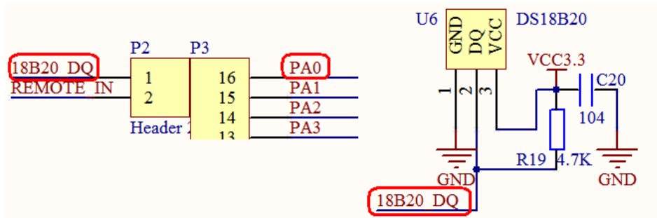
图 28.2.1 DS18B20 接口与 STM32 的连接电路图
