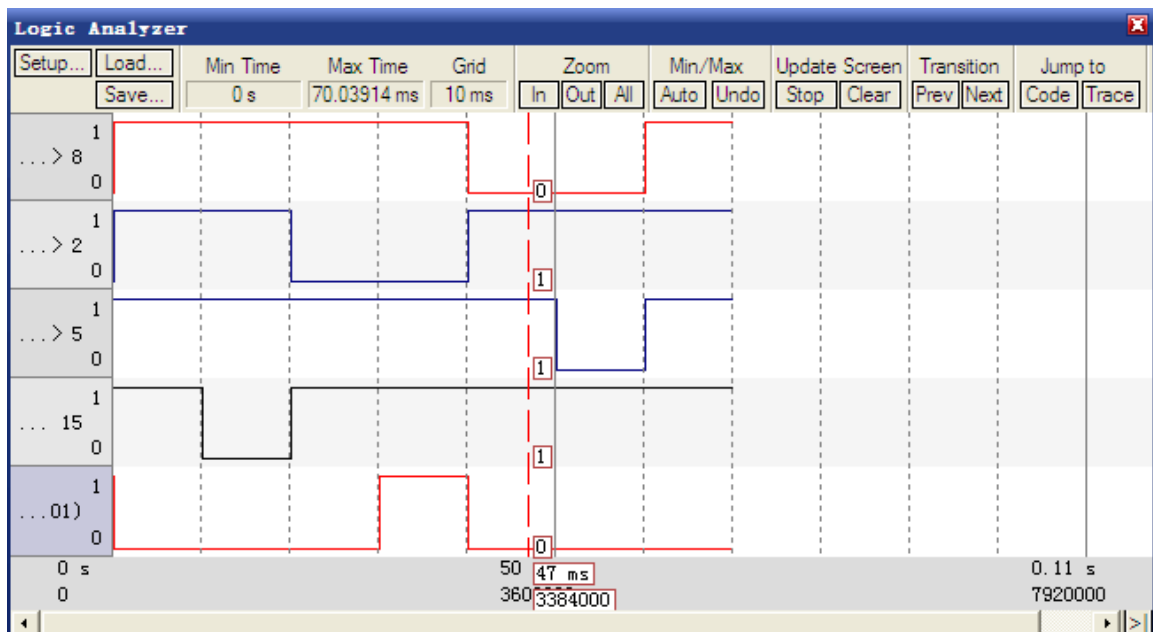
图 7.4.5 仿真波形
