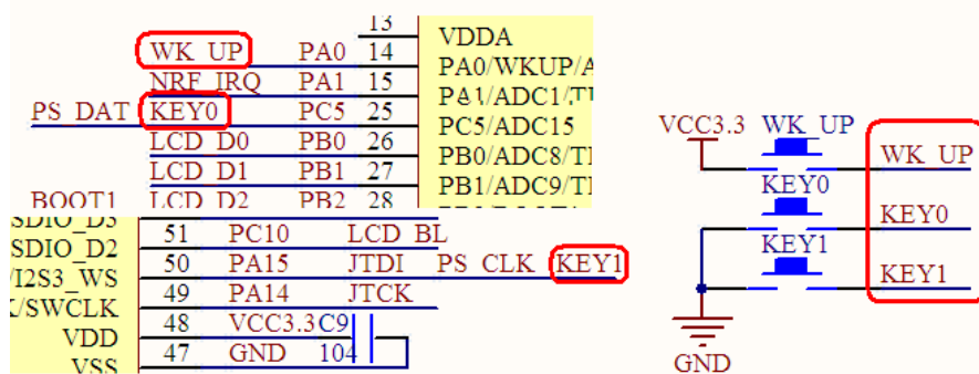
图 7.2.1 按键与 STM32 连接原理图
