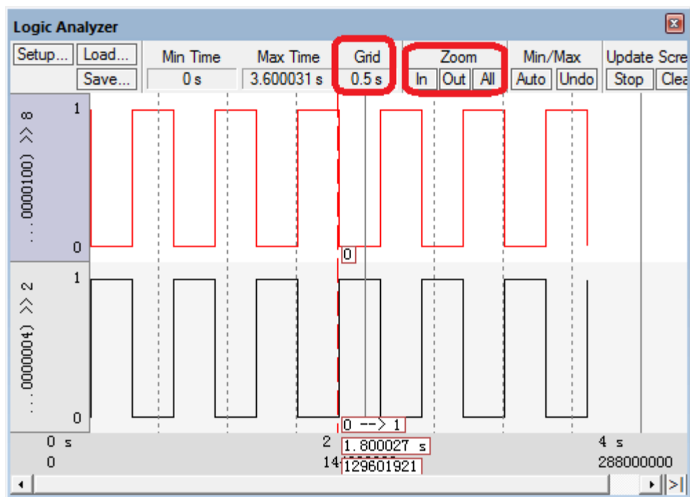
图 6.4.3 仿真波形
