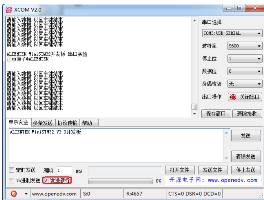
图 8.4.1 串口调试助手收到的信息
