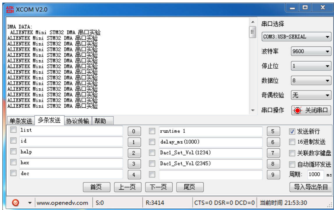
图 23.4.2 串口收到的数据内容
