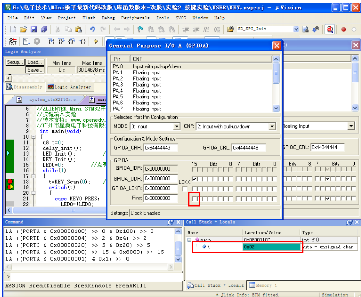
图 7.4.4 按键扫描结果
