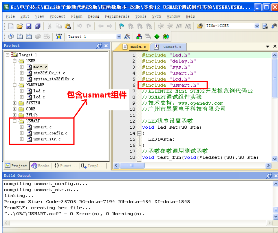
图 17.3.2 添加 USMART 组件代码
