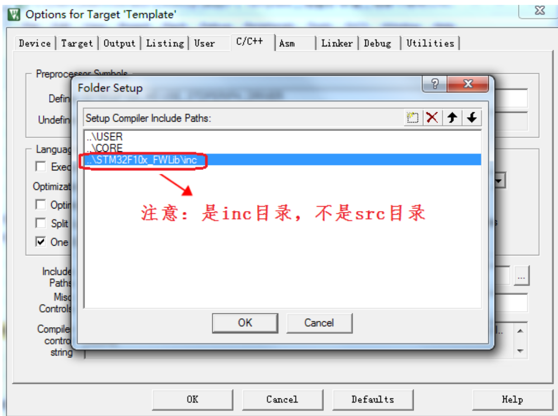
图 3.3.3.19 C/C++选项卡
