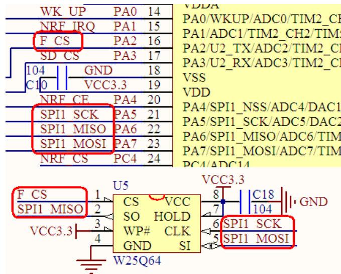
图 25.2.1 STM32 与 W25Q64 连接电路图
