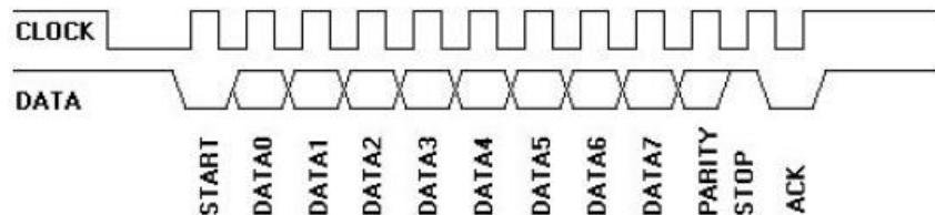
图 30.1.3 主机到设备通信时序图
