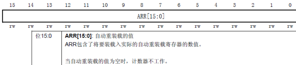
图 12.1.4 TIMx_ARR 寄存器各位描述
