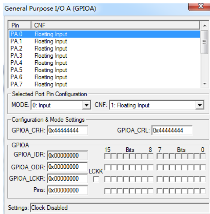
图 7.4.2 查看 GPIOA 寄存器
