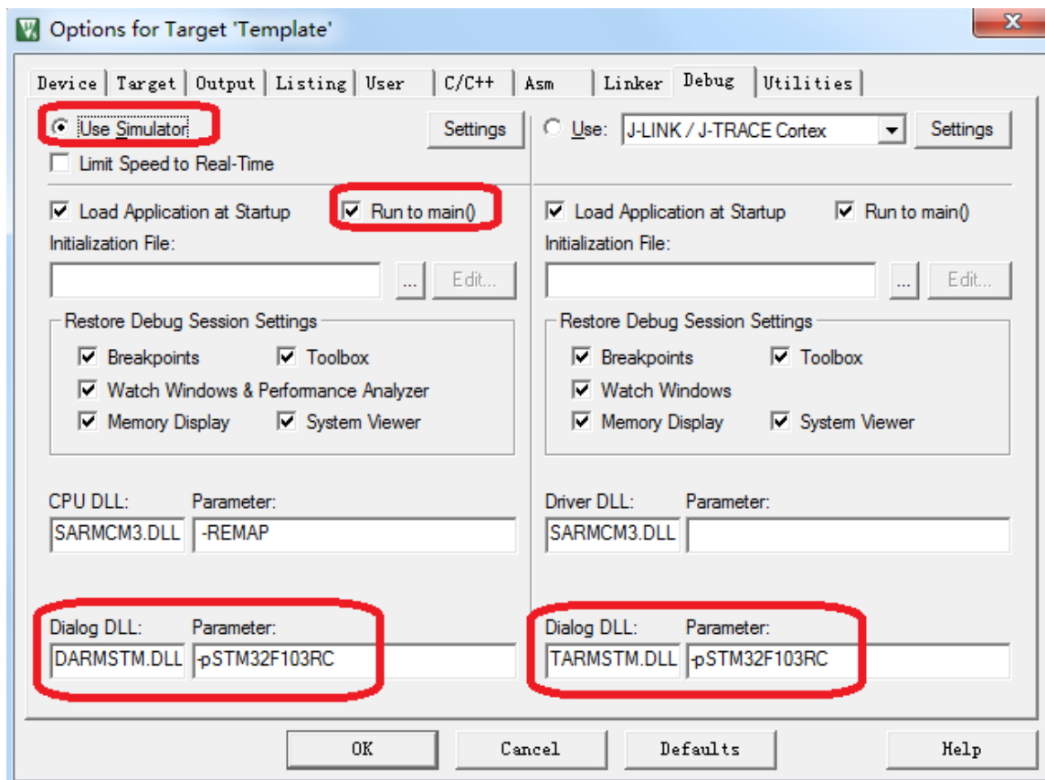
图 3.4.1.2 Debug 选项卡
