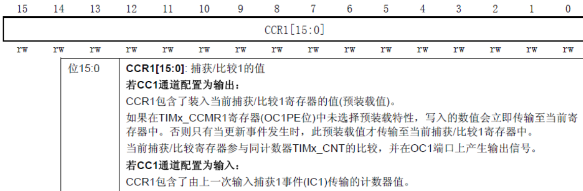
图 13.1.3 寄存器 TIMx_CCR1 各位描述
