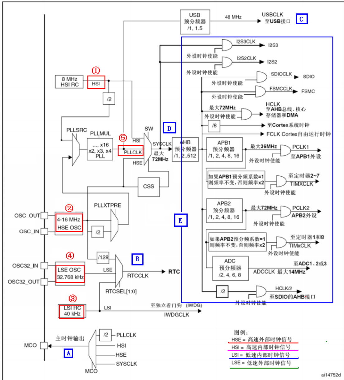
图 4.3.1 STM32 时钟系统图
