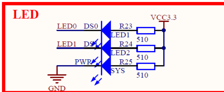
图 2.1.8.1 LED 原理图
