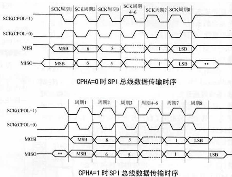
图 25.1.2 不同时钟相位下的总线传输时序（CPHA=0/1）
