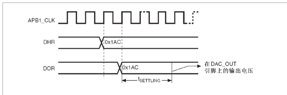
图 22.1.2 TEN=0 时 DAC 模块转换时间框图
