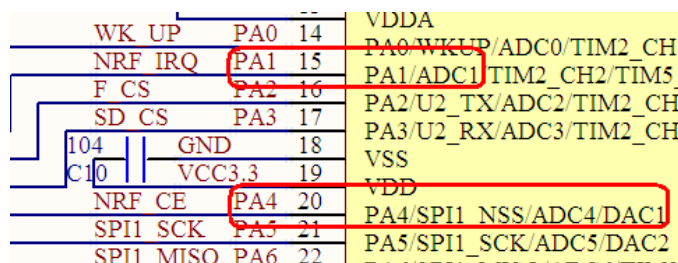
图 22.2.1 ADC、DAC 与 STM32 连接原理图
