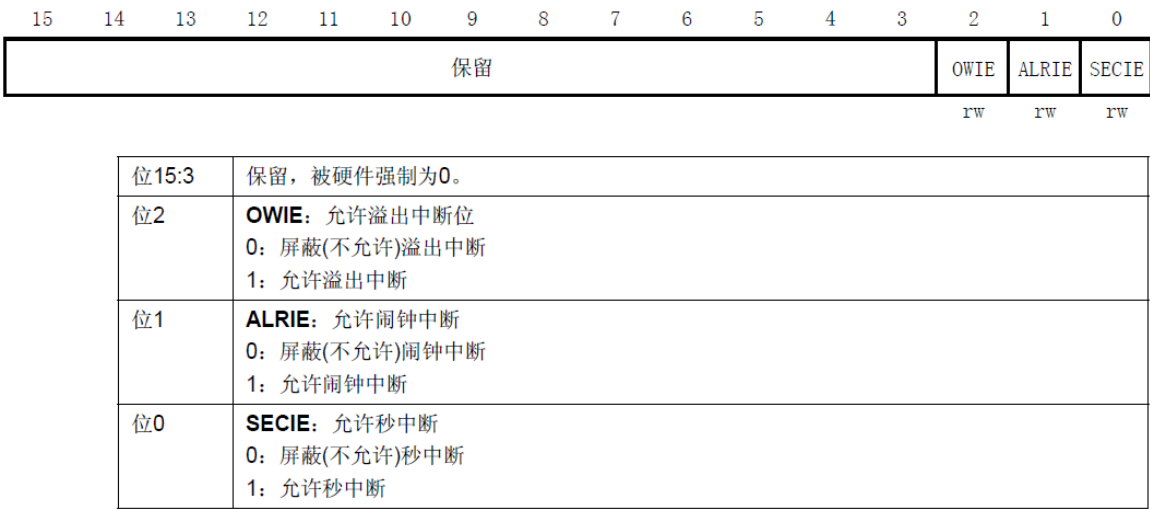
图 18.1.2 RTC_CRH 寄存器各位描述
