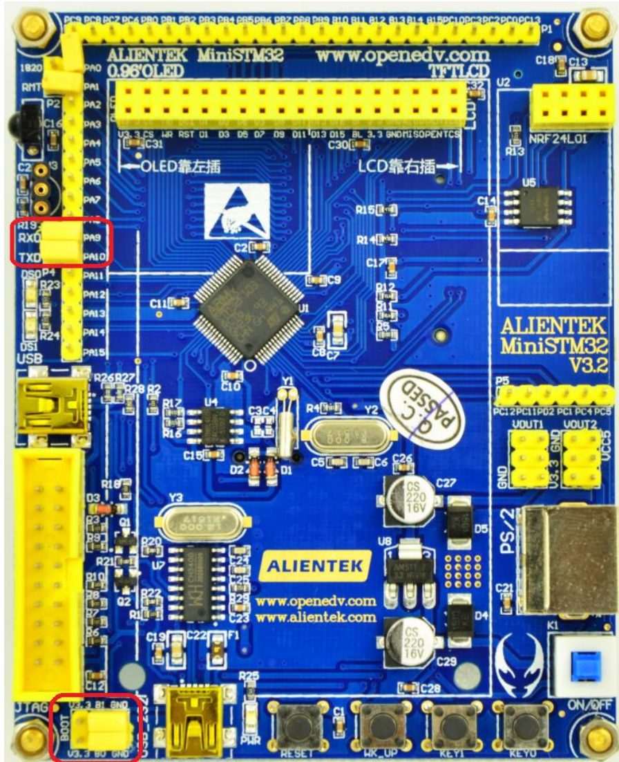
图 3.4.2.1 开发板串口下载跳线设置
