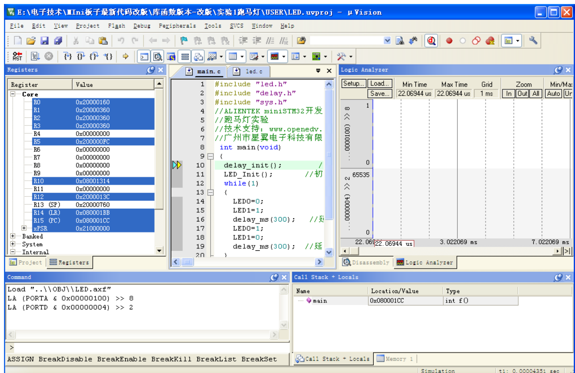
图 6.4.2 设置后的逻辑分析窗口
