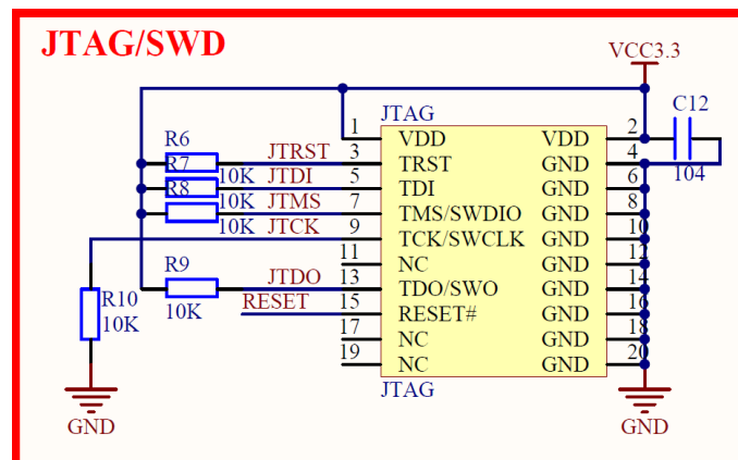
图 2.1.1.2 JTAG 原理图
