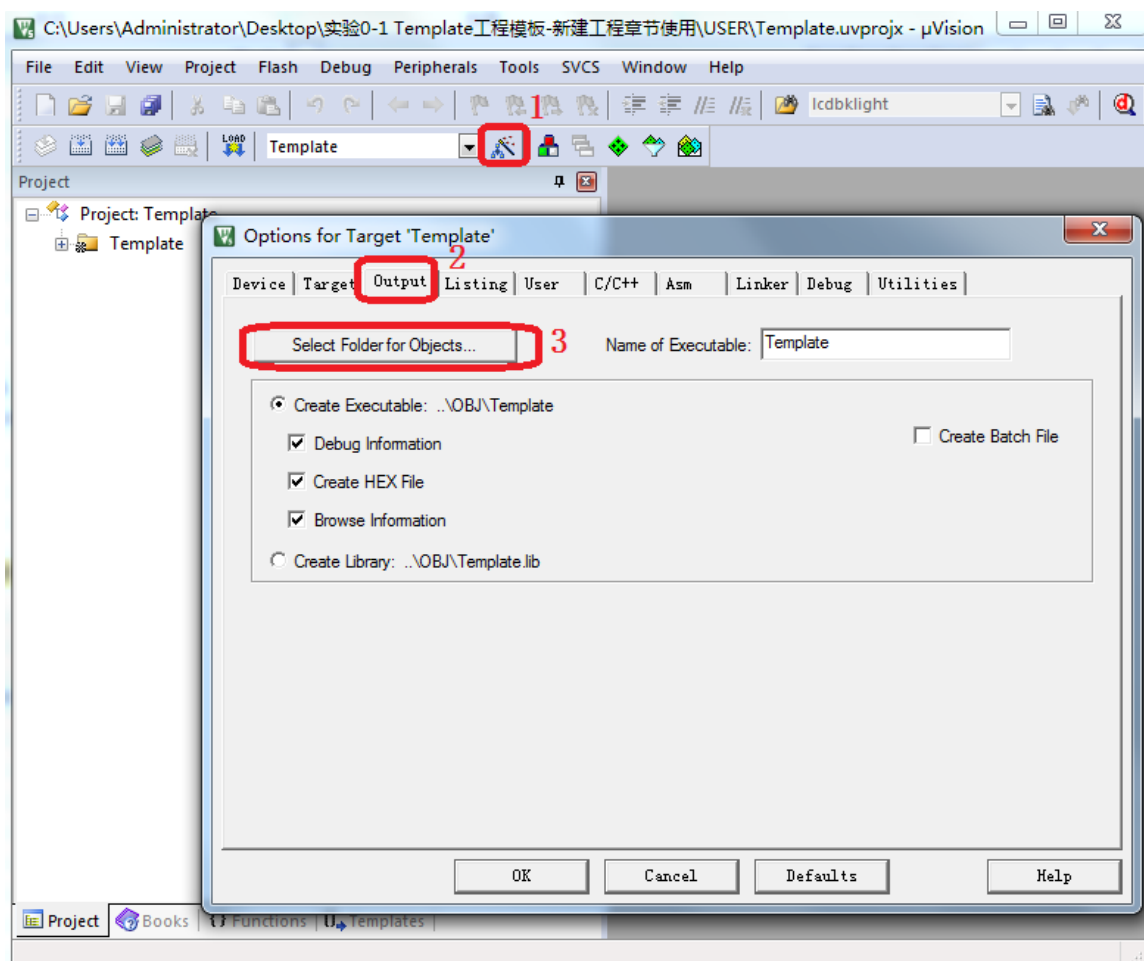
图 3.3.3.16 选择编译后的文件存放目录
