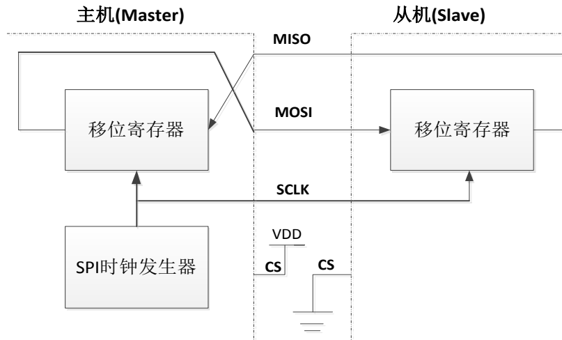
图 25.1.1 SPI 内部结构简明图
