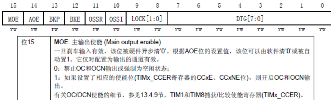
图 13.1.4 寄存器 TIMx_BDTR 各位描述
