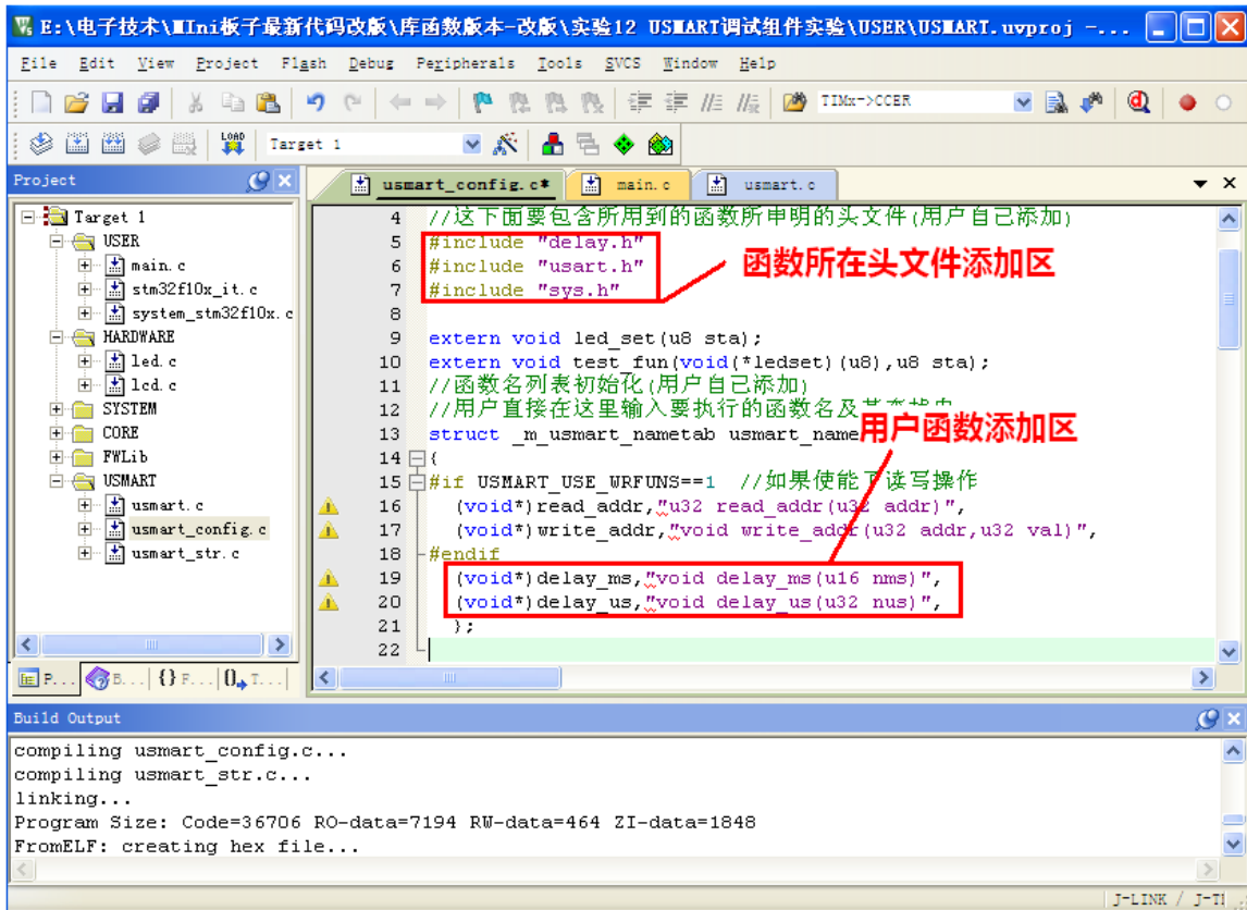
图 17.3.3 添加需要被 USMART 调用的函数
