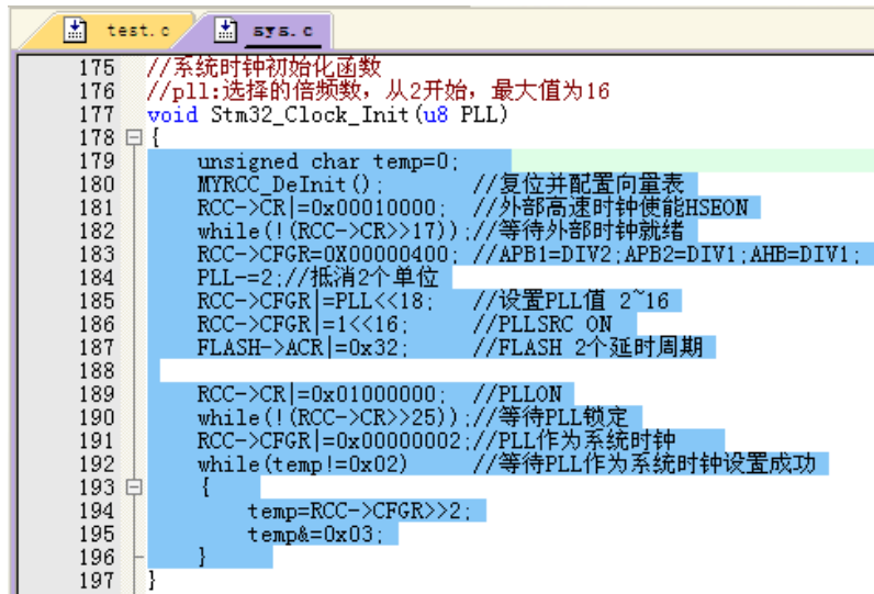
图 3.5.3.6 选中要注释的区域
