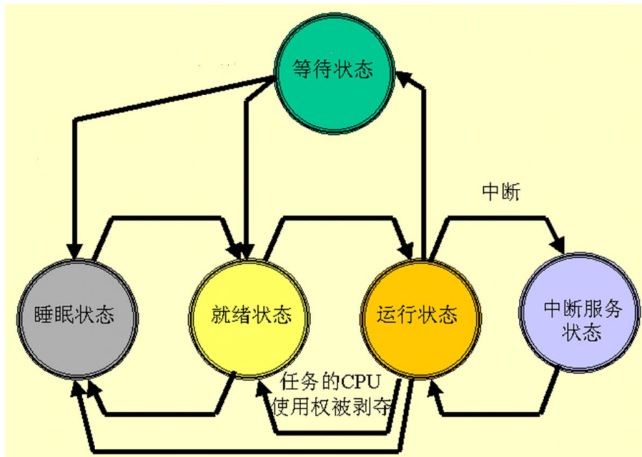
图 58.1.2 UCOSII 任务状态转换关系
