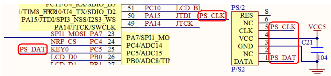
图 30.2.1 PS/2 接口与 STM32 的连接电路图
