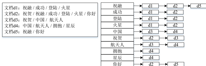
图 2 两种查找表构建策略
