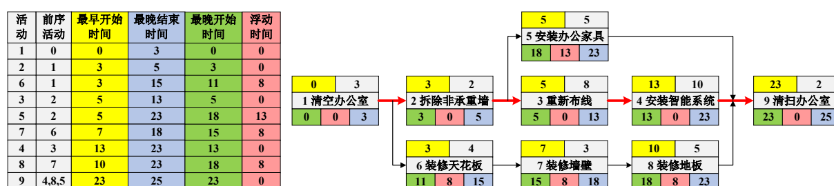
图 8 依据事件（顶点）的拓扑序列计算各项时间
