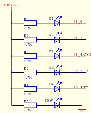
指示灯
