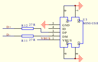
USB口
