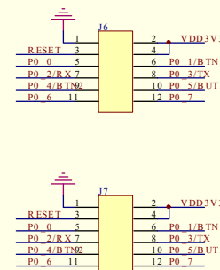
2530扩展IO口
