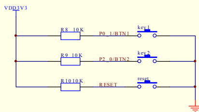
功能按键
