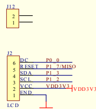
LCD接口
