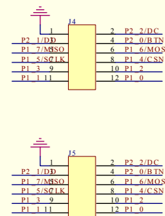
2530扩展IO口
