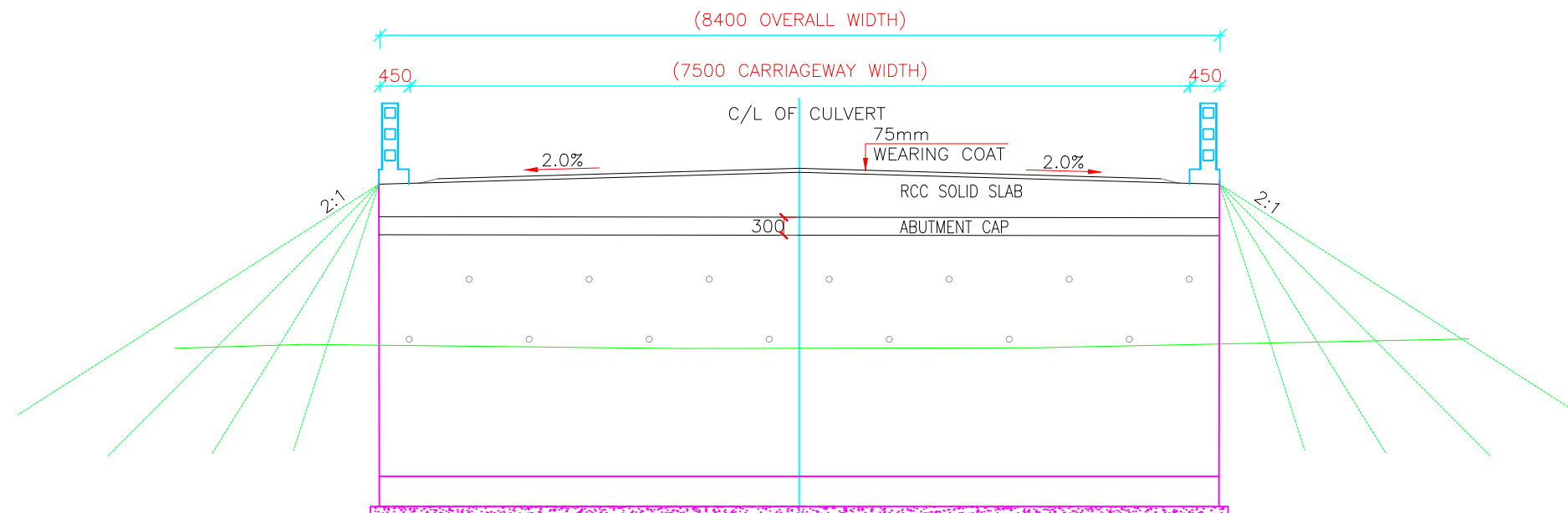
SECTION A-A
