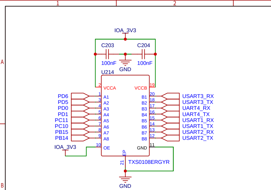
串口引脚电平转换+ESD
