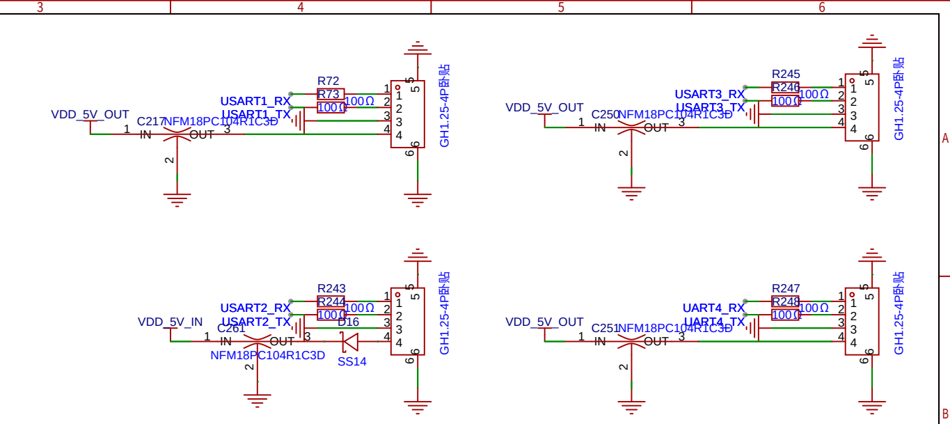
串口接口
