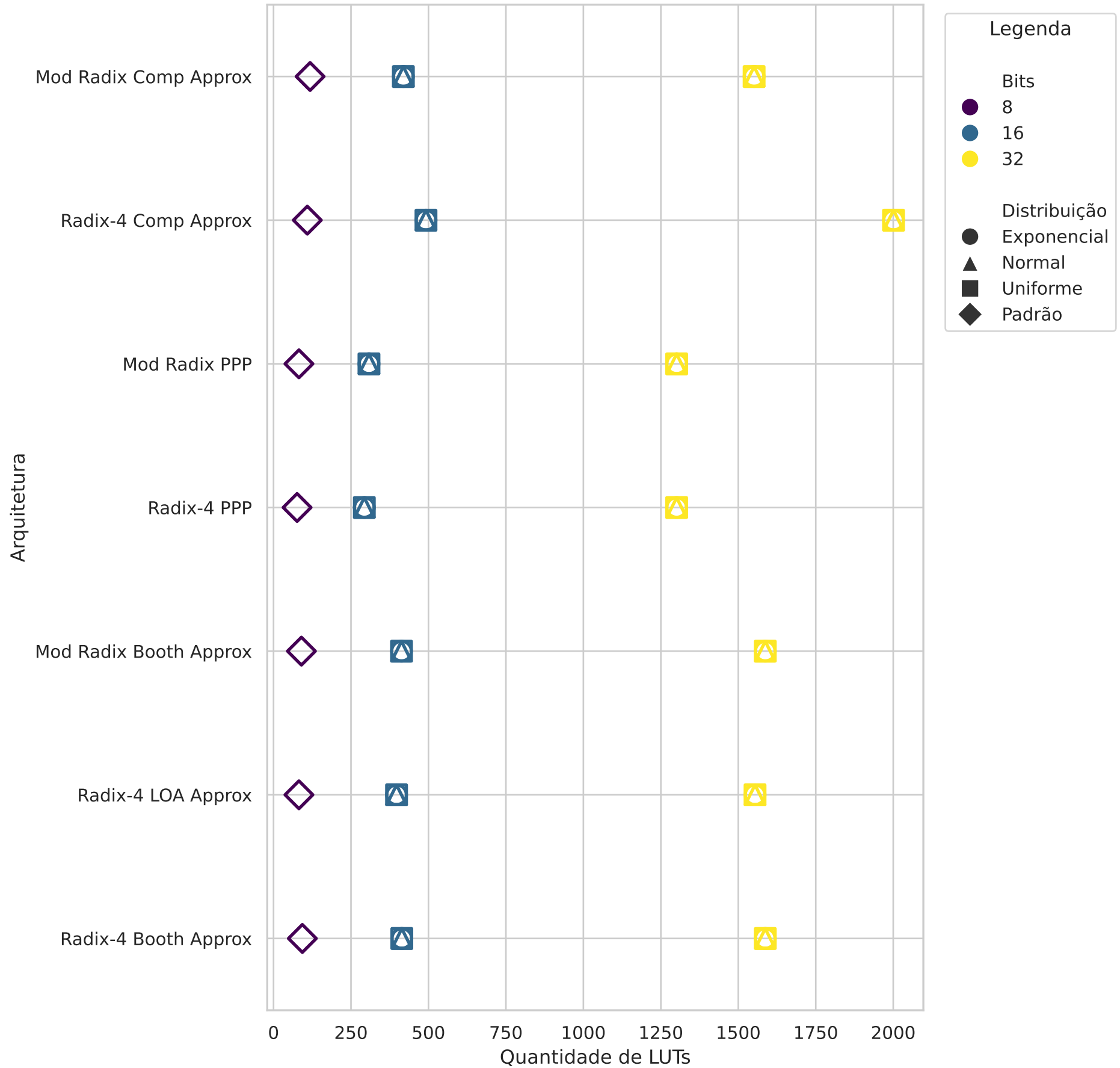
Comparação de Uso de LUTs - Aproximados
