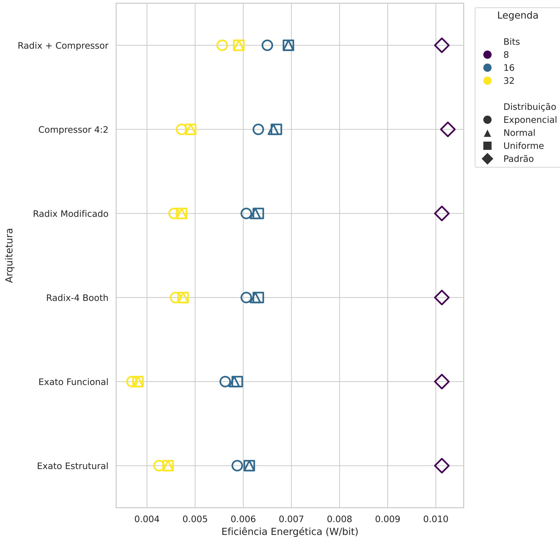
Comparação de Eficiência Energética (menor = melhor) - Exatos
