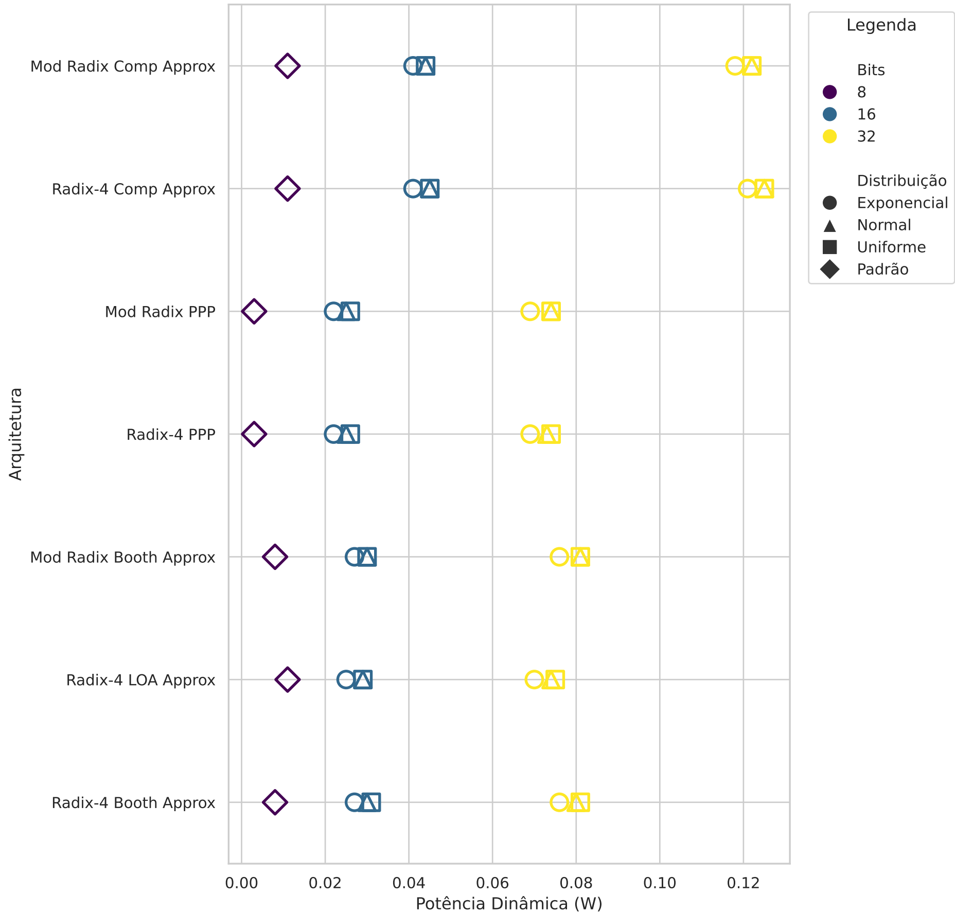
Comparação de Potência Dinâmica - Aproximados
