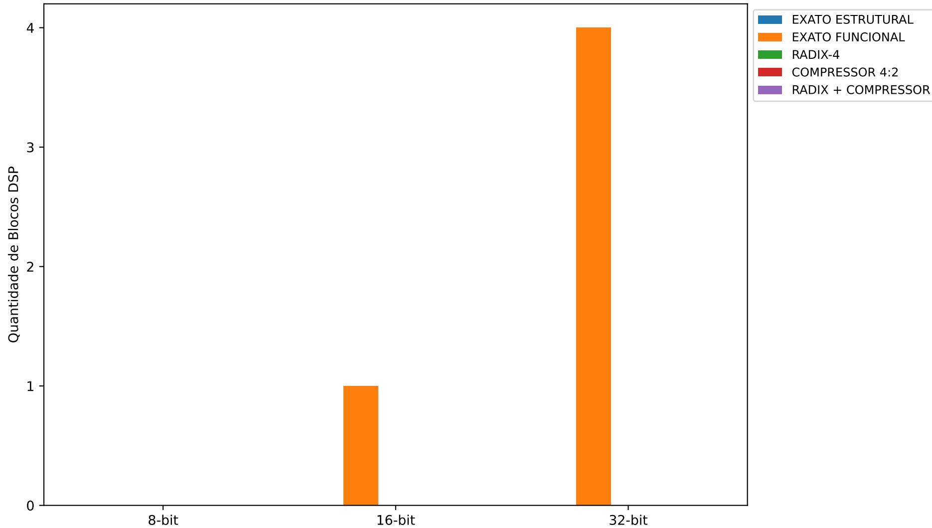
Comparação de uso de Blocos DSP
