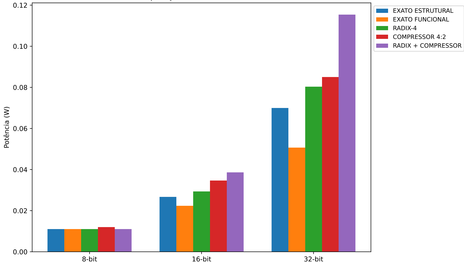
Comparação de Potência Dinâmica
