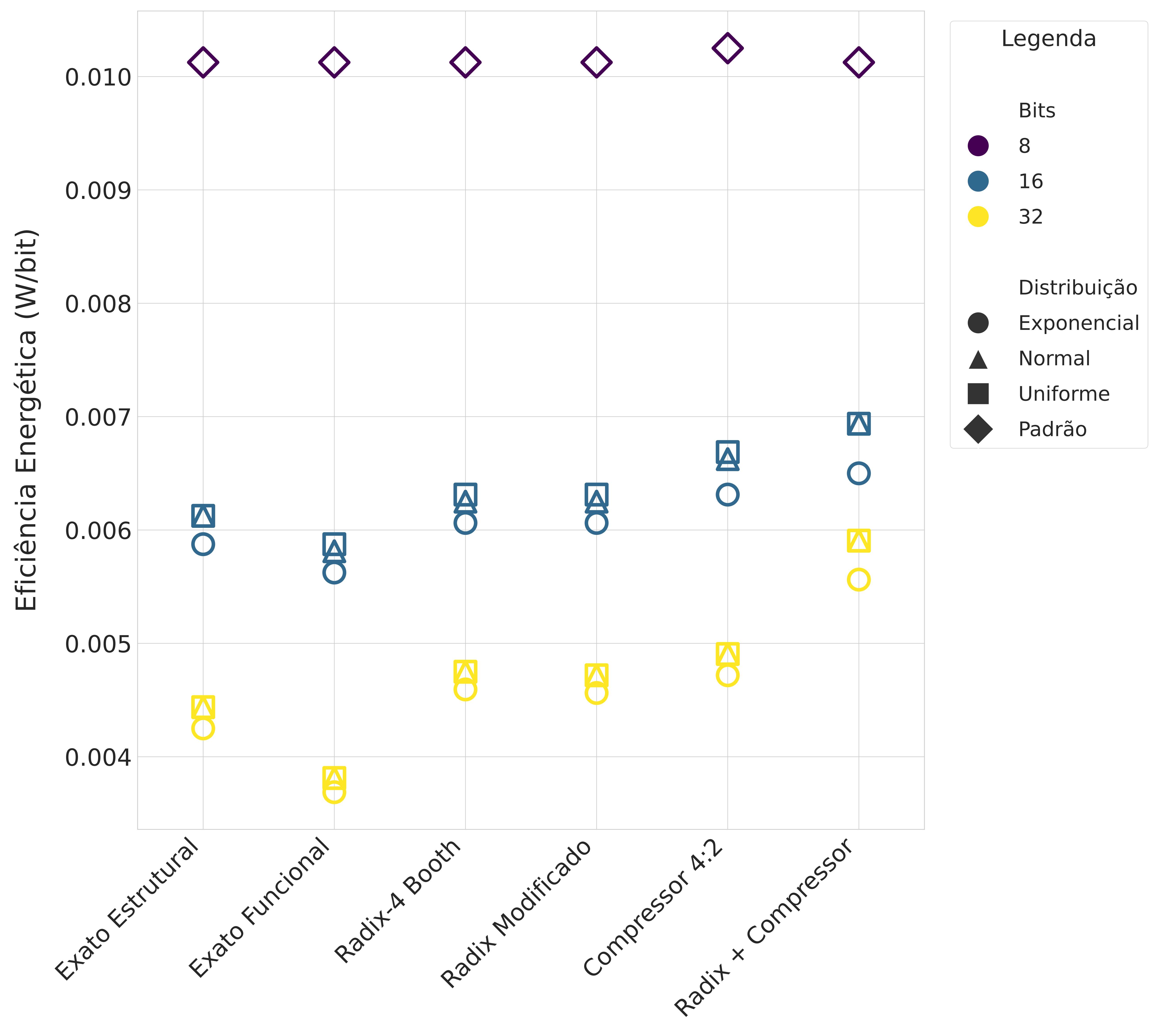
Comparação de Eficiência Energética (menor = melhor) - Exatos
