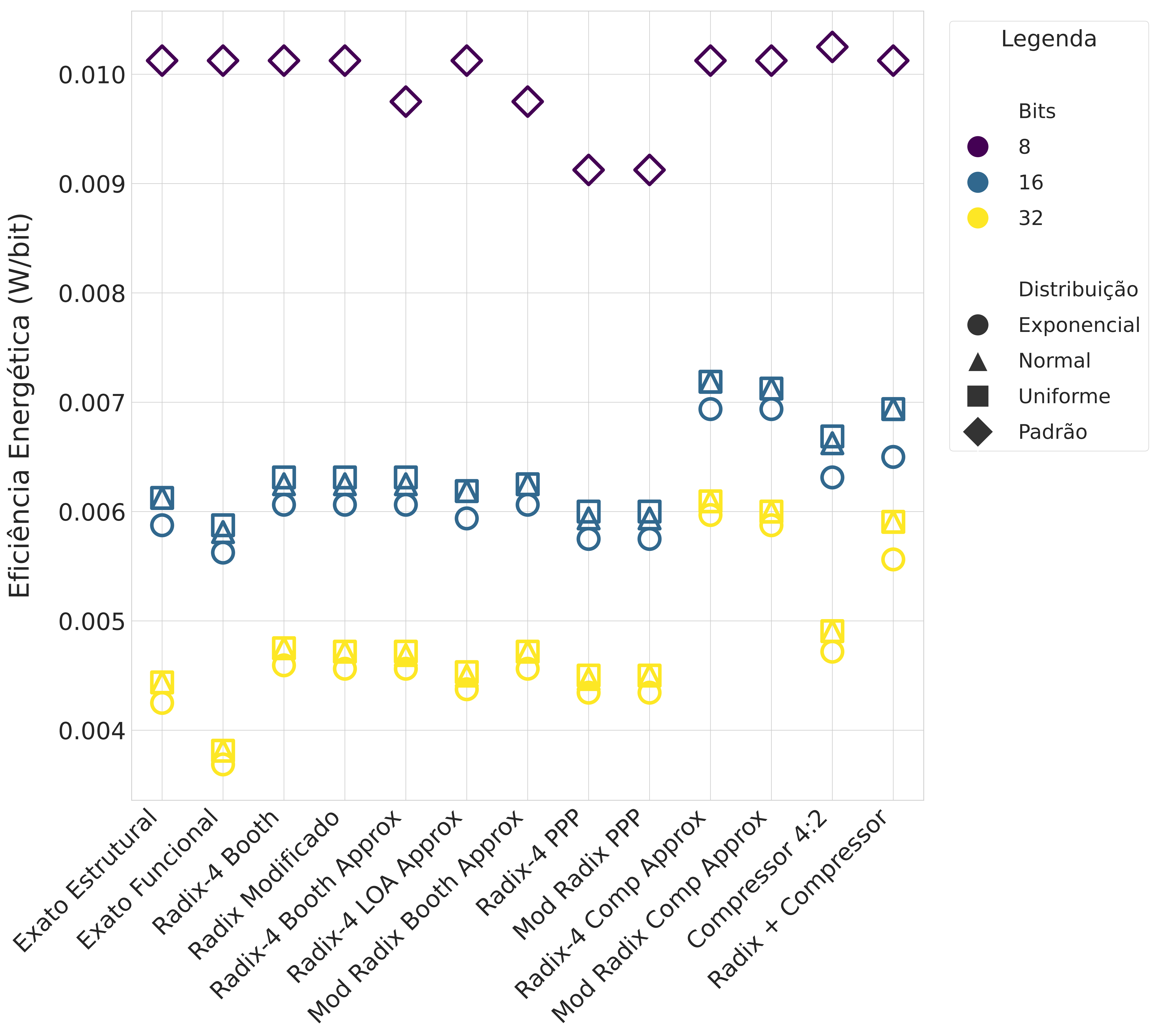
Comparação de Eficiência Energética (menor = melhor) - Todos
