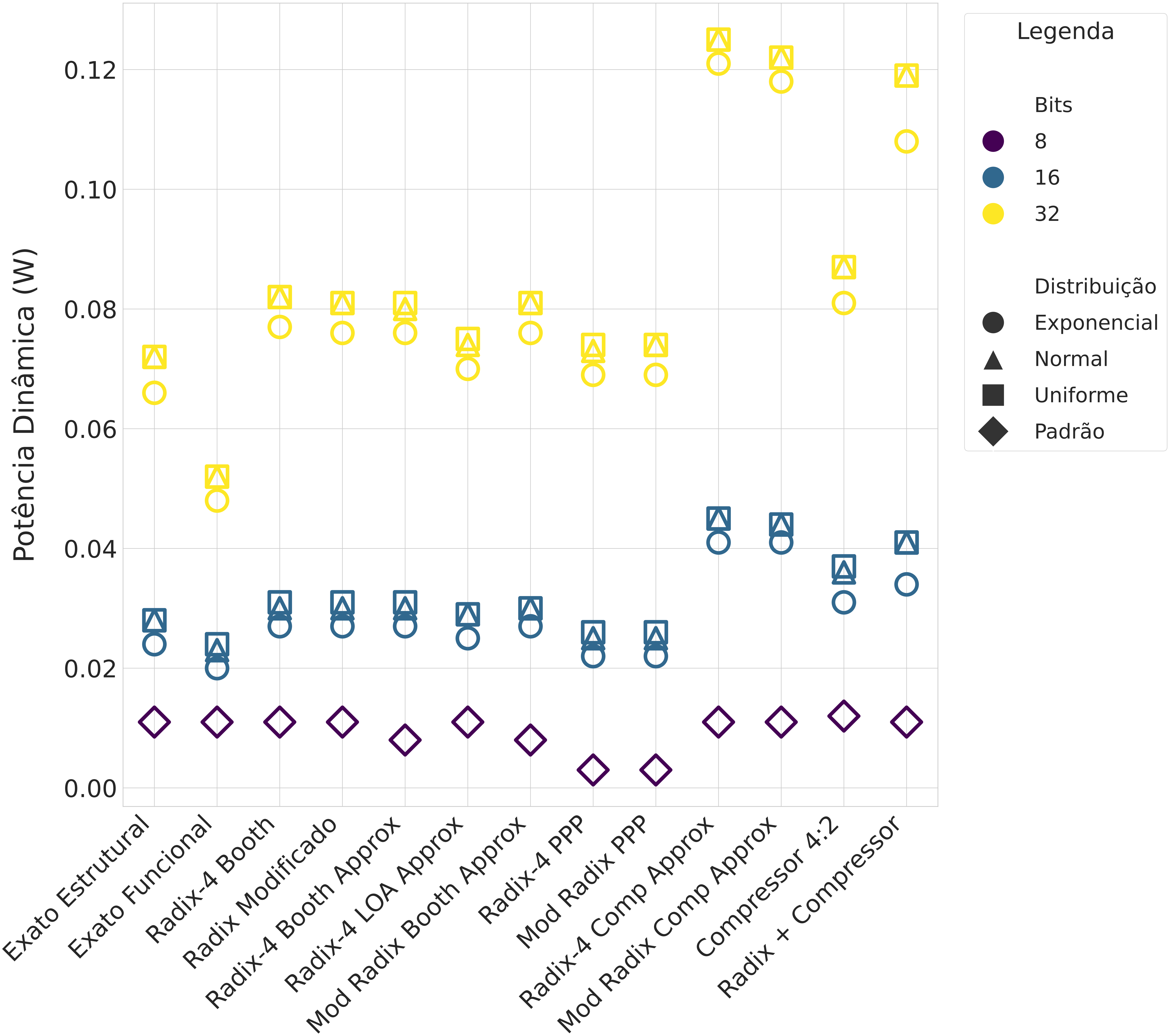
Comparação de Potência Dinâmica - Todos
