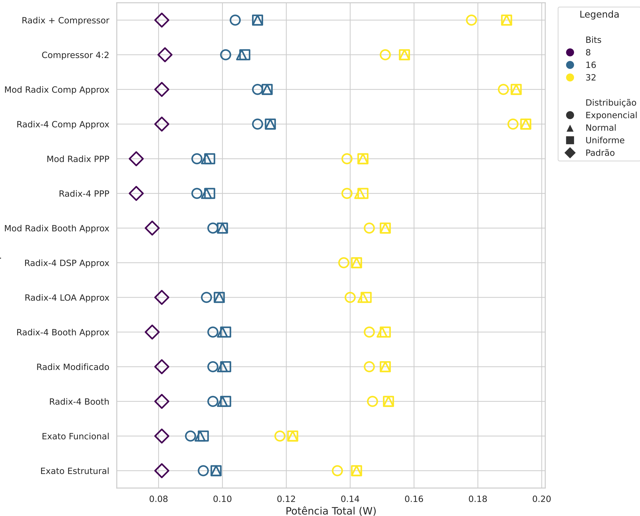
Comparação de Potência Total
