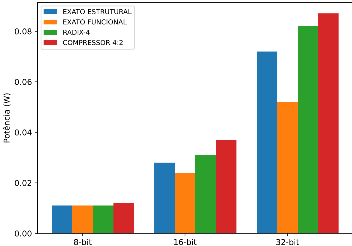
Comparação de Potência Dinâmica
